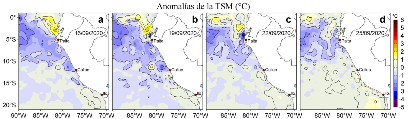
Figura 3. Anomalías de la temperatura superficial del mar (TSM, °C) para los días: a) 16, b) 19, c) 22 y d) 25 de setiembre de 2020. Las anomalías se calcularon respecto de la climatología para el periodo 2007-2016. Datos: OSTIA-UKMO-L4-GLOB-v2.0 (UK Met Office, 2012; Donlon et al, 2012). Procesamiento: LHFMAFIOF/DGIOCC.
