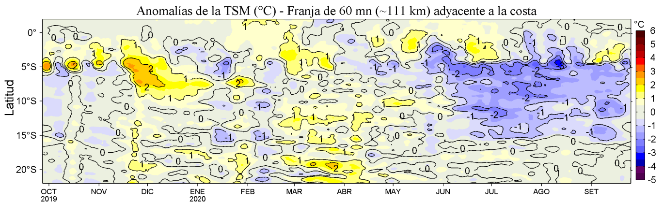
Figura 4. Variación promedio de las anomalías de la temperatura superficial del mar (TSM, °C) para una franja de 60 mn (~111 km) adyacente al litoral peruano para los últimos doce meses al 25 de setiembre de 2020. Datos: OSTIA-UKMO-L4-GLOB-v2.0 (UK Met. Office, 2012; Donlon et al, 2012) disponible en https://podaac.jpl.nasa.gov/dataset/OSTIA-UKMO-L4-GLOB-v2.0 . Las anomalías se calcularon con respecto al periodo 2007-2016. Procesamiento: LHFMAFIOF/DGIOCC.
