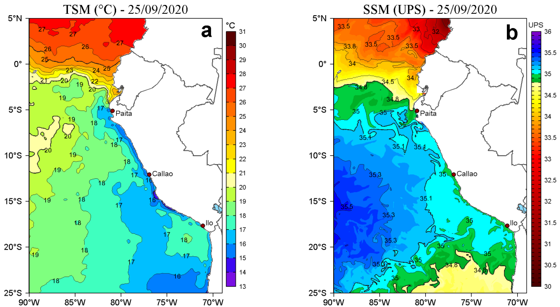
Figura 2. a) Temperatura superficial del mar (TSM, °C) y b) Salinidad superficial del mar (SSM, UPS), para el 25 de setiembre de 2020. Datos: OSTIA-UKMO-L4-GLOB-v2.0 (UK Met Office, 2012; Donlon et al, 2012) disponible en https://podaac.jpl.nasa.gov/dataset/OSTIA-UKMO-L4-GLOB-v2.0 para (a) y Hybrid Coordinate Ocean Model v. GOFS 3.1 (HYCOM; Halliwell et al., 1998; 2000; Bleck, 2001) para (b). Procesamiento: LHFMAFIOF/DGIOCC.
