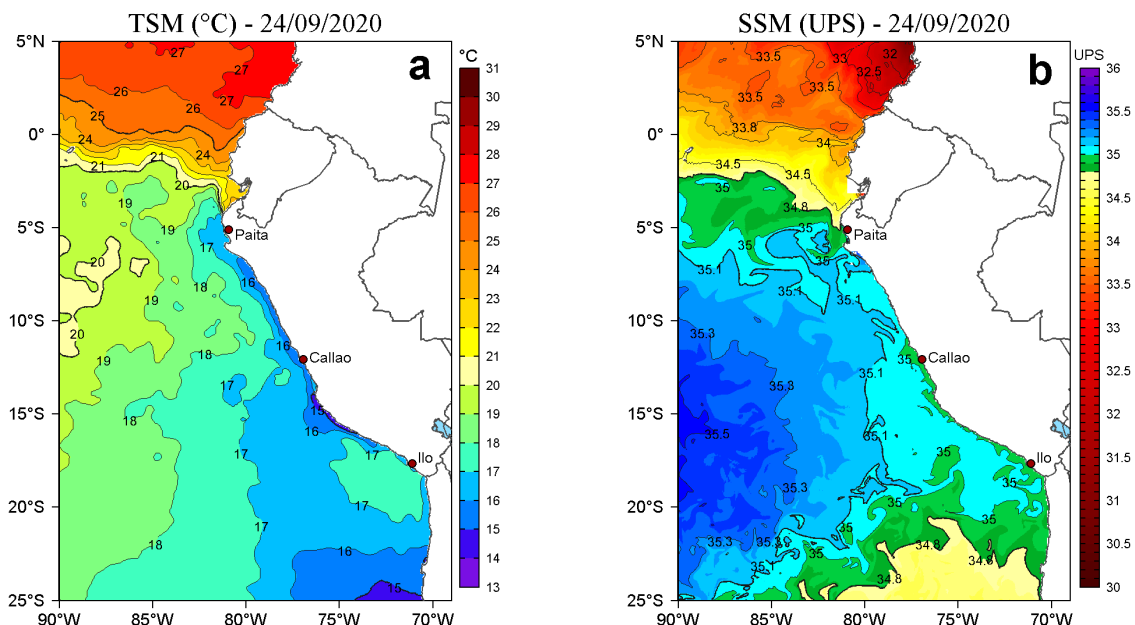
Figura 2. a) Temperatura superficial del mar (TSM, °C) y b) Salinidad superficial del mar (SSM, UPS), para el 24 de setiembre de 2020. Datos: OSTIA-UKMO-L4-GLOB-v2.0 (UK Met Office, 2012; Donlon et al, 2012) disponible en https://podaac.jpl.nasa.gov/dataset/OSTIA-UKMO-L4-GLOB-v2.0 para (a) y Hybrid Coordinate Ocean Model v. GOFS 3.1 (HYCOM; Halliwell et al., 1998; 2000; Bleck, 2001) para (b). Procesamiento: LHFMAFIOF/DGIOCC.
