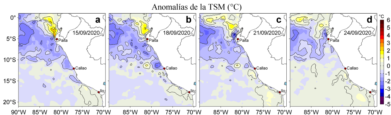
Figura 3. Anomalías de la temperatura superficial del mar (TSM, °C) para los días: a) 15, b) 18, c) 21 y d) 24 de setiembre de 2020. Las anomalías se calcularon respecto de la climatología para el periodo 2007-2016. Datos: OSTIA-UKMO-L4-GLOB-v2.0 (UK Met Office, 2012; Donlon et al, 2012). Procesamiento: LHFMAFIOF/DGIOCC.
