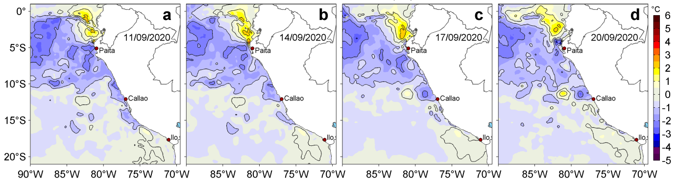
Figura 3. Anomalías de la temperatura superficial del mar (TSM, °C) para los días: a) 11, b) 14, c) 17 y d) 20 de setiembre de 2020. Las anomalías se calcularon respecto de la climatología para el periodo 2007-2016. Datos: OSTIA-UKMO-L4-GLOB-v2.0 (UK Met Office, 2012; Donlon et al, 2012). Procesamiento: LHF/AFIOF/DGIOCC.
