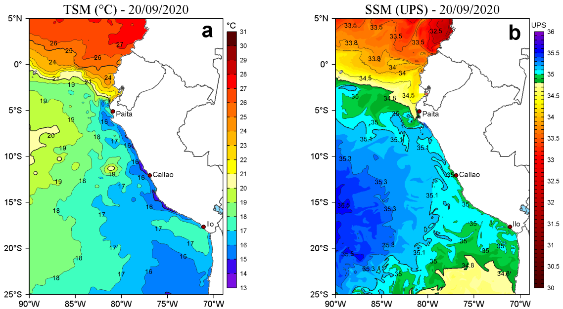
Figura 2. a) Temperatura superficial del mar (TSM, °C) y b) Salinidad superficial del mar (SSM, UPS), para el 20 de setiembre de 2020. Datos: OSTIA-UKMO-L4-GLOB-v2.0 (UK Met Office, 2012; Donlon et al, 2012) disponible en https://podaac.jpl.nasa.gov/dataset/OSTIA-UKMO-L4-GLOB-v2.0 para (a) y Hybrid Coordinate Ocean Model v. GOFS 3.1 (HYCOM; Halliwell et al., 1998; 2000; Bleck, 2001) para (b). Procesamiento: LHF/AFIOF/DGIOCC.
