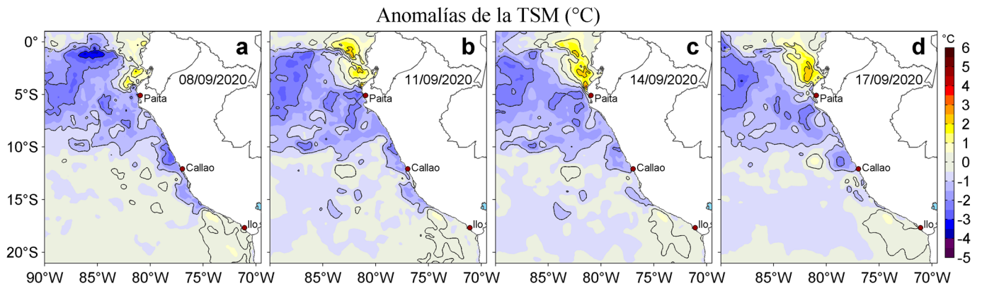
Figura 3. Anomalías de la temperatura superficial del mar (TSM, °C) para los días: a) 08, b) 11, c) 14 y d) 17 de setiembre de 2020. Las anomalías se calcularon respecto de la climatología para el periodo 2007-2016. Datos: OSTIA-UKMO-L4-GLOB-v2.0 (UK Met Office, 2012; Donlon et al, 2012). Procesamiento: LHF/AFIOF/DGIOCC.
