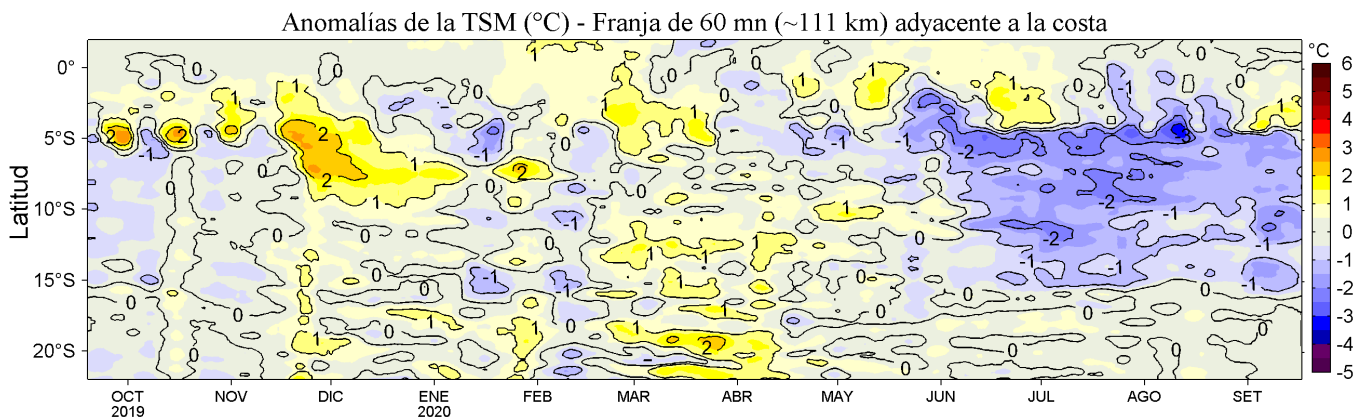
Figura 4. Variación promedio de las anomalías de la temperatura superficial del mar (TSM, °C) para una franja de 60 mn (~111 km) adyacente al litoral peruano para los últimos doce meses al 17 de setiembre de 2020. Datos: OSTIA-UKMO-L4-GLOB-v2.0 (UK Met. Office, 2012; Donlon et al, 2012) disponible en https://podaac.jpl.nasa.gov/dataset/OSTIA-UKMO-L4-GLOB-v2.0 . Las anomalías se calcularon con respecto al periodo 2007-2016. Procesamiento: LHF/AFIOF/DGIOCC.
