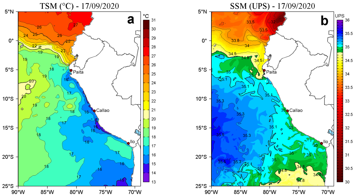
Figura 2. a) Temperatura superficial del mar (TSM, °C) y b) Salinidad superficial del mar (SSM, UPS), para el 17 de setiembre de 2020. Datos: OSTIA-UKMO-L4-GLOB-v2.0 (UK Met Office, 2012; Donlon et al, 2012) disponible en https://podaac.jpl.nasa.gov/dataset/OSTIA-UKMO-L4-GLOB-v2.0 para (a) y Hybrid Coordinate Ocean Model v. GOFS 3.1 (HYCOM; Halliwell et al., 1998; 2000; Bleck, 2001) para (b). Procesamiento: LHF/AFIOF/DGIOCC.
