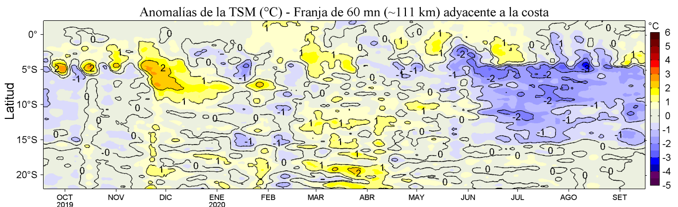
Figura 4. Variación promedio de las anomalías de la temperatura superficial del mar (TSM, °C) para una franja de 60 mn (~111 km) adyacente al litoral peruano para los últimos doce meses al 16 de setiembre de 2020. Datos: OSTIA-UKMO-L4-GLOB-v2.0 (UK Met. Office, 2012; Donlon et al, 2012) disponible en https://podaac.jpl.nasa.gov/dataset/OSTIA-UKMO-L4-GLOB-v2.0 . Las anomalías se calcularon con respecto al periodo 2007-2016. Procesamiento: LHF/AFIOF/DGIOCC.
