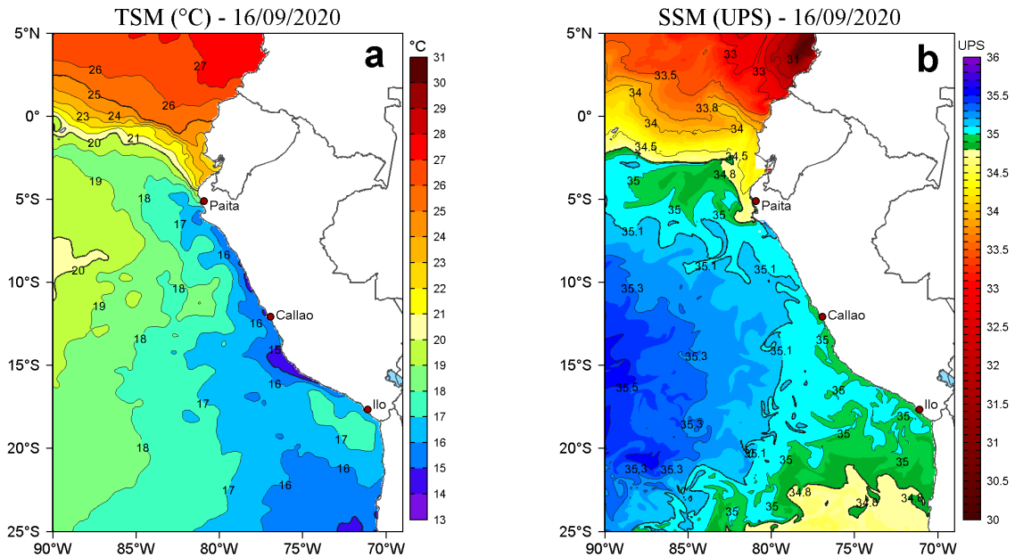
Figura 2. a) Temperatura superficial del mar (TSM, °C) y b) Salinidad superficial del mar (SSM, UPS), para el 16 de setiembre de 2020. Datos: OSTIA-UKMO-L4-GLOB-v2.0 (UK Met Office, 2012; Donlon et al, 2012) disponible en https://podaac.jpl.nasa.gov/dataset/OSTIA-UKMO-L4-GLOB-v2.0 para (a) y Hybrid Coordinate Ocean Model v. GOFS 3.1 (HYCOM; Halliwell et al., 1998; 2000; Bleck, 2001) para (b). Procesamiento: LHF/AFIOF/DGIOCC.
