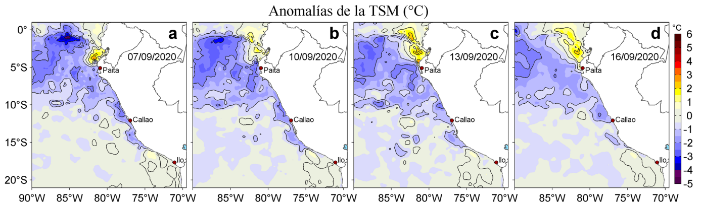
Figura 3. Anomalías de la temperatura superficial del mar (TSM, °C) para los días: a) 07, b) 10, c) 13 y d) 16 de setiembre de 2020. Las anomalías se calcularon respecto de la climatología para el periodo 2007-2016. Datos: OSTIA-UKMO-L4-GLOB-v2.0 (UK Met Office, 2012; Donlon et al, 2012). Procesamiento: LHF/AFIOF/DGIOCC.
