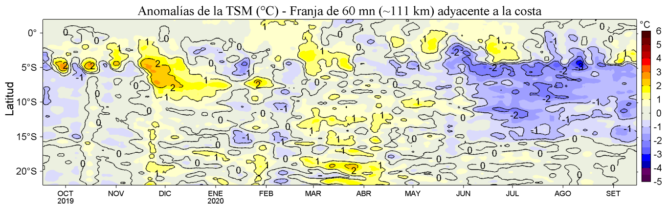
Figura 4. Variación promedio de las anomalías de la temperatura superficial del mar (TSM, °C) para una franja de 60 mn (~111 km) adyacente al litoral peruano para los últimos doce meses al 15 de setiembre de 2020. Datos: OSTIA-UKMO-L4-GLOB-v2.0 (UK Met. Office, 2012; Donlon et al, 2012) disponible en https://podaac.jpl.nasa.gov/dataset/OSTIA-UKMO-L4-GLOB-v2.0 . Las anomalías se calcularon con respecto al periodo 2007-2016. Procesamiento: LHF/AFIOF/DGIOCC.
