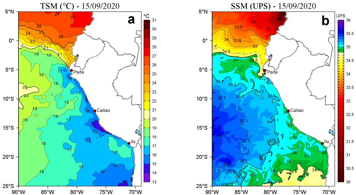
Figura 2. a) Temperatura superficial del mar (TSM, °C) y b) Salinidad superficial del mar (SSM, UPS), para el 15 de setiembre de 2020. Datos: OSTIA-UKMO-L4-GLOB-v2.0 (UK Met Office, 2012; Donlon et al, 2012) disponible en https://podaac.jpl.nasa.gov/dataset/OSTIA-UKMO-L4-GLOB-v2.0 para (a) y Hybrid Coordinate Ocean Model v. GOFS 3.1 (HYCOM; Halliwell et al., 1998; 2000; Bleck, 2001) para (b). Procesamiento: LHF/AFIOF/DGIOCC.
