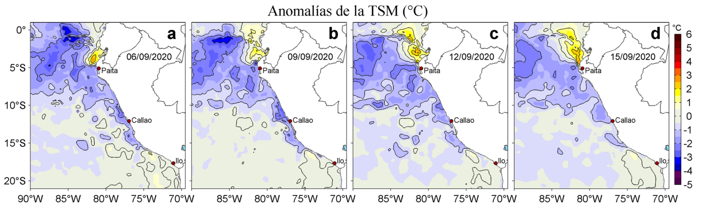
Figura 3. Anomalías de la temperatura superficial del mar (TSM, °C) para los días: a) 06, b) 09, c) 12 y d) 15 de setiembre de 2020. Las anomalías se calcularon respecto de la climatología para el periodo 2007-2016. Datos: OSTIA-UKMO-L4-GLOB-v2.0 (UK Met Office, 2012; Donlon et al, 2012). Procesamiento: LHF/AFIOF/DGIOCC.
