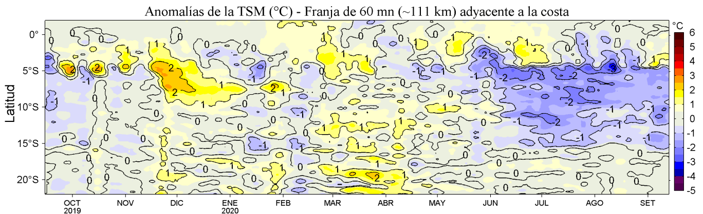
Figura 4. Variación promedio de las anomalías de la temperatura superficial del mar (TSM, °C) para una franja de 60 mn (~111 km) adyacente al litoral peruano para los últimos doce meses al 13 de setiembre de 2020. Datos: OSTIA-UKMO-L4-GLOB-v2.0 (UK Met. Office, 2012; Donlon et al, 2012) disponible en https://podaac.jpl.nasa.gov/dataset/OSTIA-UKMO-L4-GLOB-v2.0 . Las anomalías se calcularon con respecto al periodo 2007-2016. Procesamiento: LHF/AFIOF/DGIOCC.
