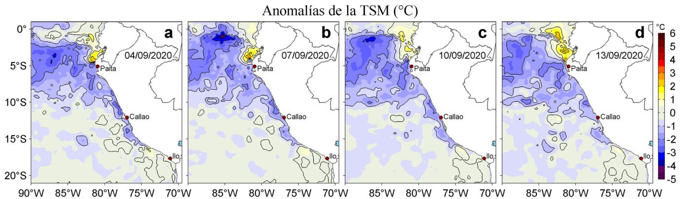
Figura 3. Anomalías de la temperatura superficial del mar (TSM, °C) para los días: a) 04, b) 07, c) 10 y d) 13 de setiembre de 2020. Las anomalías se calcularon respecto de la climatología para el periodo 2007-2016. Datos: OSTIA-UKMO-L4-GLOB-v2.0 (UK Met Office, 2012; Donlon et al, 2012). Procesamiento: LHF/AFIOF/DGIOCC.
