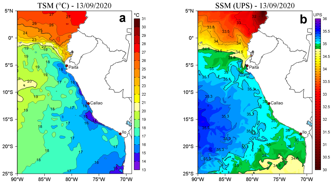
Figura 2. a) Temperatura superficial del mar (TSM, °C) y b) Salinidad superficial del mar (SSM, UPS), para el 13 de setiembre de 2020. Datos: OSTIA-UKMO-L4-GLOB-v2.0 (UK Met Office, 2012; Donlon et al, 2012) disponible en https://podaac.jpl.nasa.gov/dataset/OSTIA-UKMO-L4-GLOB-v2.0 para (a) y Hybrid Coordinate Ocean Model v. GOFS 3.1 (HYCOM; Halliwell et al., 1998; 2000; Bleck, 2001) para (b). Procesamiento: LHF/AFIOF/DGIOCC.
