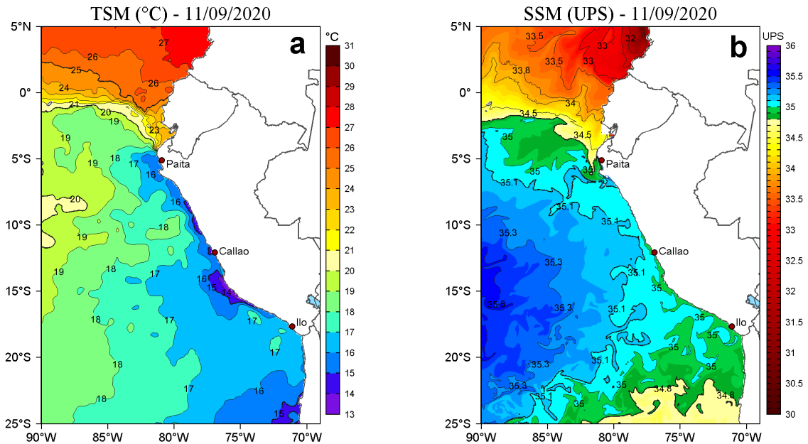
Figura 2. a) Temperatura superficial del mar (TSM, °C) y b) Salinidad superficial del mar (SSM, UPS), para el 11 de setiembre de 2020. Datos: OSTIA-UKMO-L4-GLOB-v2.0 (UK Met Office, 2012; Donlon et al, 2012) disponible en https://podaac.jpl.nasa.gov/dataset/OSTIA-UKMO-L4-GLOB-v2.0 para (a) y Hybrid Coordinate Ocean Model v. GOFS 3.1 (HYCOM; Halliwell et al., 1998; 2000; Bleck, 2001) para (b). Procesamiento: LHF/AFIOF/DGIOCC.
