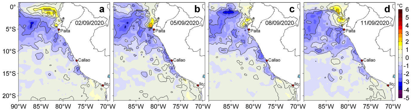
Figura 3. Anomalías de la temperatura superficial del mar (TSM, °C) para los días: a) 02, b) 05, c) 08 y d) 11 de setiembre de 2020. Las anomalías se calcularon respecto de la climatología para el periodo 2007-2016. Datos: OSTIA-UKMO-L4-GLOB-v2.0 (UK Met Office, 2012; Donlon et al, 2012). Procesamiento: LHF/AFIOF/DGIOCC.
