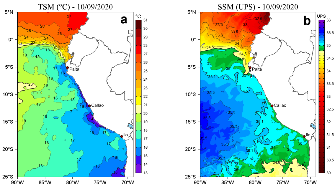
Figura 2. a) Temperatura superficial del mar (TSM, °C) y b) Salinidad superficial del mar (SSM, UPS), para el 10 de setiembre de 2020. Datos: OSTIA-UKMO-L4-GLOB-v2.0 (UK Met Office, 2012; Donlon et al, 2012) disponible en https://podaac.jpl.nasa.gov/dataset/OSTIA-UKMO-L4-GLOB-v2.0 para (a) y Hybrid Coordinate Ocean Model v. GOFS 3.1 (HYCOM; Halliwell et al., 1998; 2000; Bleck, 2001) para (b). Procesamiento: LHF/AFIOF/DGIOCC.
