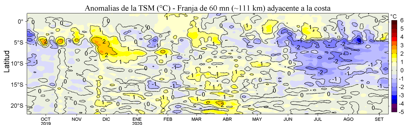
Figura 4. Variación promedio de las anomalías de la temperatura superficial del mar (TSM, °C) para una franja de 60 mn (~111 km) adyacente al litoral peruano para los últimos doce meses al 10 de setiembre de 2020. Datos: OSTIA-UKMO-L4-GLOB-v2.0 (UK Met. Office, 2012; Donlon et al, 2012) disponible en https://podaac.jpl.nasa.gov/dataset/OSTIA-UKMO-L4-GLOB-v2.0 . Las anomalías se calcularon con respecto al periodo 2007-2016. Procesamiento: LHF/AFIOF/DGIOCC.
