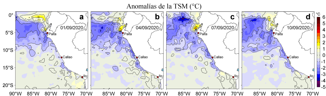
Figura 3. Anomalías de la temperatura superficial del mar (TSM, °C) para los días: a) 01, b) 04, c) 07 y d) 10 de setiembre de 2020. Las anomalías se calcularon respecto de la climatología para el periodo 2007-2016. Datos: OSTIA-UKMO-L4-GLOB-v2.0 (UK Met Office, 2012; Donlon et al, 2012). Procesamiento: LHF/AFIOF/DGIOCC.
