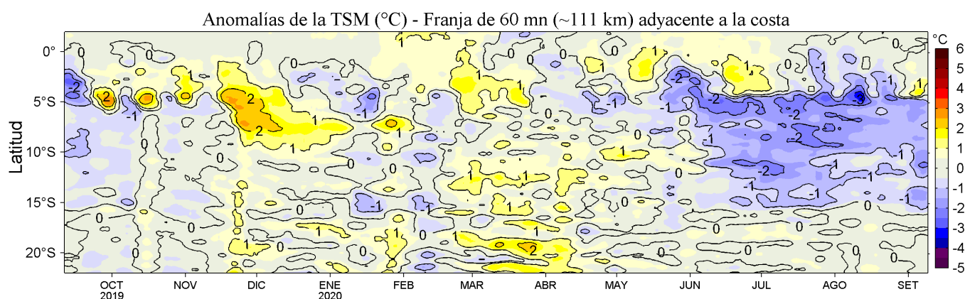
Figura 4. Variación promedio de las anomalías de la temperatura superficial del mar (TSM, °C) para una franja de 60 mn (~111 km) adyacente al litoral peruano para los últimos doce meses al 09 de setiembre de 2020. Datos: OSTIA-UKMO-L4-GLOB-v2.0 (UK Met. Office, 2012; Donlon et al, 2012) disponible en https://podaac.jpl.nasa.gov/dataset/OSTIA-UKMO-L4-GLOB-v2.0 . Las anomalías se calcularon con respecto al periodo 2007-2016. Procesamiento: LHFH/AFIOF/DGIOCC.
