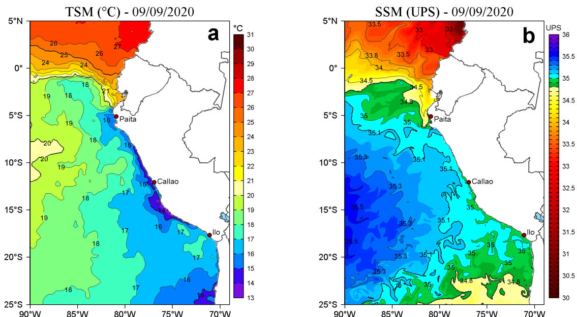
Figura 2. a) Temperatura superficial del mar (TSM, °C) y b) Salinidad superficial del mar (SSM, UPS) para el 09 de setiembre de 2020. Datos: OSTIA-UKMO-L4-GLOB-v2.0 (UK Met Office, 2012; Donlon et al, 2012) disponible en https://podaac.jpl.nasa.gov/dataset/OSTIA-UKMO-L4-GLOB-v2.0 para (a) y Hybrid Coordinate Ocean Model v. GOFS 3.1 (HYCOM; Halliwell et al., 1998; 2000; Bleck, 2001) para (b). Procesamiento: LHFH/AFIOF/DGIOCC.
