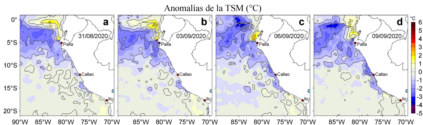
Figura 3. Anomalías de la temperatura superficial del mar (TSM, °C) para los días: a) 31 de agosto, b) 03, c) 06 y d) 09 de setiembre de 2020. Las anomalías se calcularon respecto de la climatología para el periodo 2007-2016. Datos: OSTIA-UKMO-L4-GLOB-v2.0 (UK Met Office, 2012; Donlon et al, 2012). Procesamiento: LHFH/AFIOF/DGIOCC.
