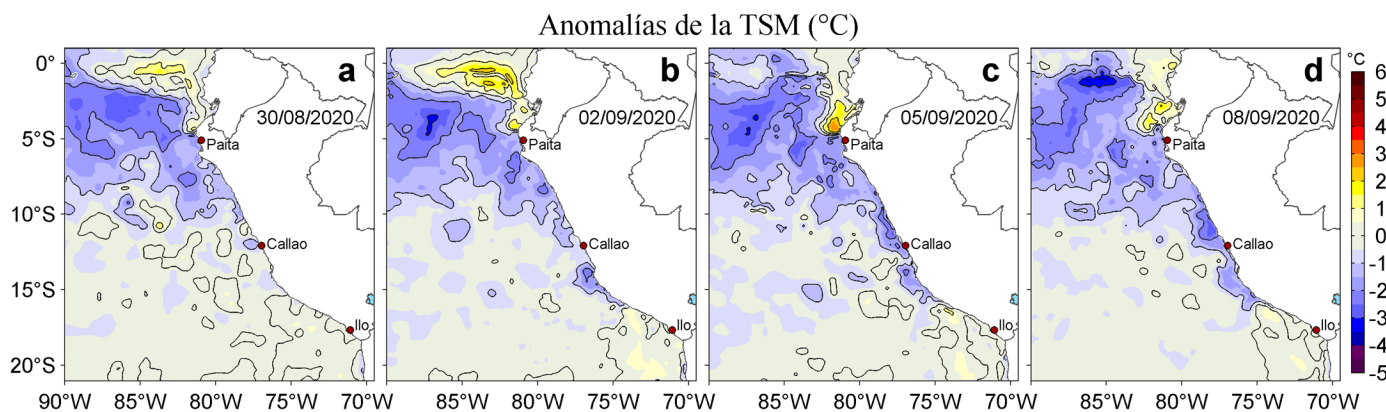
Figura 3. Anomalías de la temperatura superficial del mar (TSM, °C) para los días: a) 30 de agosto, b) 02, c) 05 y d) 08 de setiembre de 2020. Las anomalías se calcularon respecto de la climatología para el periodo 2007-2016. Datos: OSTIA-UKMO-L4-GLOB-v2.0 (UK Met Office, 2012; Donlon et al, 2012). Procesamiento: LHF/AFIOF/DGIOCC.
