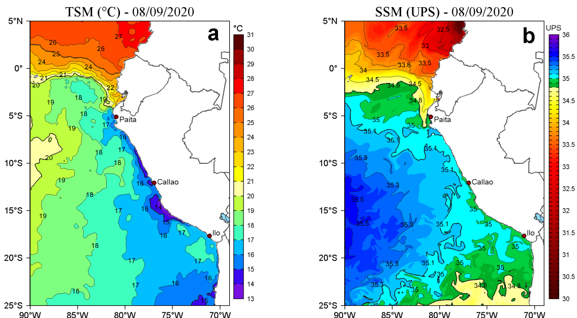
Figura 2. a) Temperatura superficial del mar (TSM, °C) y b) Salinidad superficial del mar (SSM, UPS), para el 08 de setiembre de 2020. Datos: OSTIA-UKMO-L4-GLOB-v2.0 (UK Met Office, 2012; Donlon et al, 2012) disponible en https://podaac.jpl.nasa.gov/dataset/OSTIA-UKMO-L4-GLOB-v2.0 para (a) y Hybrid Coordinate Ocean Model v. GOFS 3.1 (HYCOM; Halliwell et al., 1998; 2000; Bleck, 2001) para (b). Procesamiento: LHF/AFIOF/DGIOCC.
