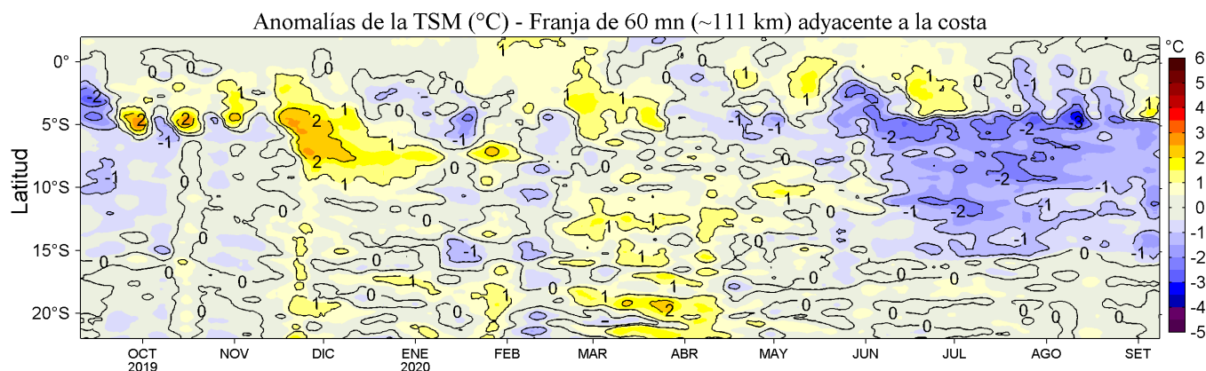
Figura 4. Variación promedio de las anomalías de la temperatura superficial del mar (TSM, °C) para una franja de 60 mn (~111 km) adyacente al litoral peruano para los últimos doce meses al 08 de setiembre de 2020. Datos: OSTIA-UKMO-L4-GLOB-v2.0 (UK Met. Office, 2012; Donlon et al, 2012) disponible en https://podaac.jpl.nasa.gov/dataset/OSTIA-UKMO-L4-GLOB-v2.0 . Las anomalías se calcularon con respecto al periodo 2007-2016. Procesamiento: LHF/AFIOF/DGIOCC.
