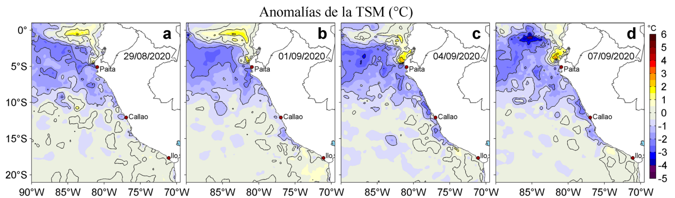
Figura 3. Anomalías de la temperatura superficial del mar (TSM, °C) para los días: a) 29 de agosto, b) 01, c) 04 y d) 07 de setiembre de 2020. Las anomalías se calcularon respecto de la climatología para el periodo 2007-2016. Datos: OSTIA-UKMO-L4-GLOB-v2.0 (UK Met Office, 2012; Donlon et al, 2012). Procesamiento: LHF/AFIOF/DGIOCC.
