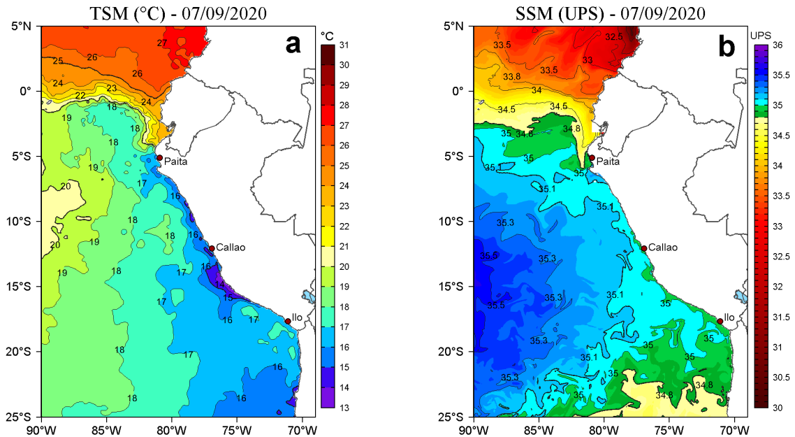
Figura 2. a) Temperatura superficial del mar (TSM, °C) y b) Salinidad superficial del mar (SSM, UPS), para el 07 de setiembre de 2020. Datos: OSTIA-UKMO-L4-GLOB-v2.0 (UK Met Office, 2012; Donlon et al, 2012) disponible en https://podaac.jpl.nasa.gov/dataset/OSTIA-UKMO-L4-GLOB-v2.0 para (a) y Hybrid Coordinate Ocean Model v. GOFS 3.1 (HYCOM; Halliwell et al., 1998; 2000; Bleck, 2001) para (b). Procesamiento: LHF/AFIOF/DGIOCC.
