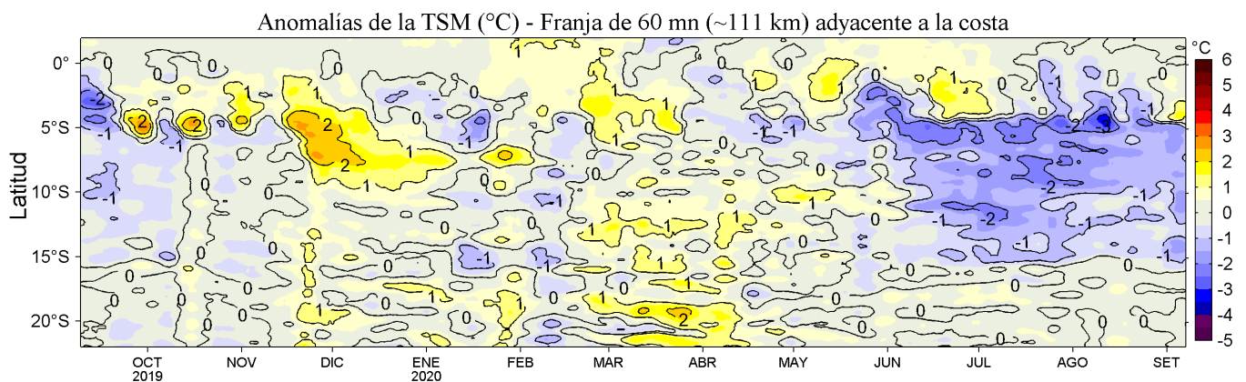
Figura 4. Variación promedio de las anomalías de la temperatura superficial del mar (TSM, °C) para una franja de 60 mn (~111 km) adyacente al litoral peruano para los últimos doce meses al 07 de setiembre de 2020. Datos: OSTIA-UKMO-L4-GLOB-v2.0 (UK Met. Office, 2012; Donlon et al, 2012) disponible en https://podaac.jpl.nasa.gov/dataset/OSTIA-UKMO-L4-GLOB-v2.0 . Las anomalías se calcularon con respecto al periodo 2007-2016. Procesamiento: LHF/AFIOF/DGIOCC.
