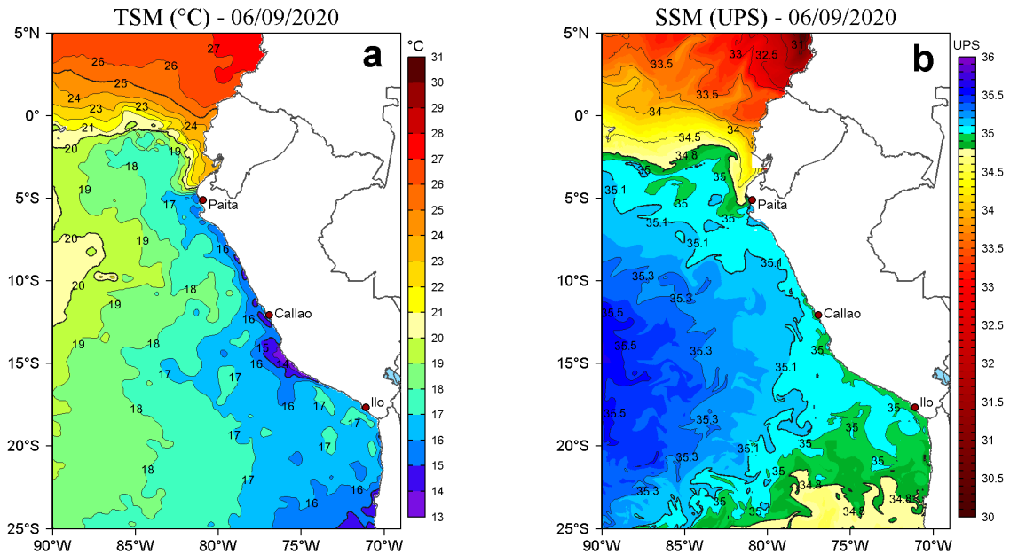
Figura 2. a) Temperatura superficial del mar (TSM, °C) y b) Salinidad superficial del mar (SSM, UPS), para el 06 de setiembre de 2020. Datos: OSTIA-UKMO-L4-GLOB-v2.0 (UK Met Office, 2012; Donlon et al, 2012) disponible en https://podaac.jpl.nasa.gov/dataset/OSTIA-UKMO-L4-GLOB-v2.0 para (a) y Hybrid Coordinate Ocean Model v. GOFS 3.1 (HYCOM; Halliwell et al., 1998; 2000; Bleck, 2001) para (b). Procesamiento: LHFMAFIOF/DGIOCC.
