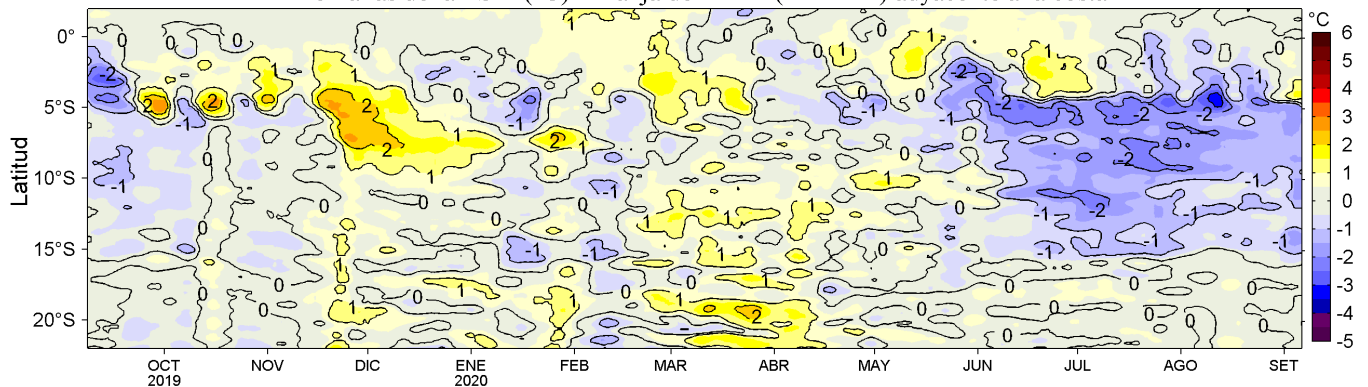
Figura 4. Variación promedio de las anomalías de la temperatura superficial del mar (TSM, °C) para una franja de 60 mn (~111 km) adyacente al litoral peruano para los últimos doce meses al 06 de setiembre de 2020. Datos: OSTIA-UKMO-L4-GLOB-v2.0 (UK Met. Office, 2012; Donlon et al, 2012) disponible en https://podaac.jpl.nasa.gov/dataset/OSTIA-UKMO-L4-GLOB-v2.0 . Las anomalías se calcularon con respecto al periodo 2007-2016. Procesamiento: LHFMAFIOF/DGIOCC.
