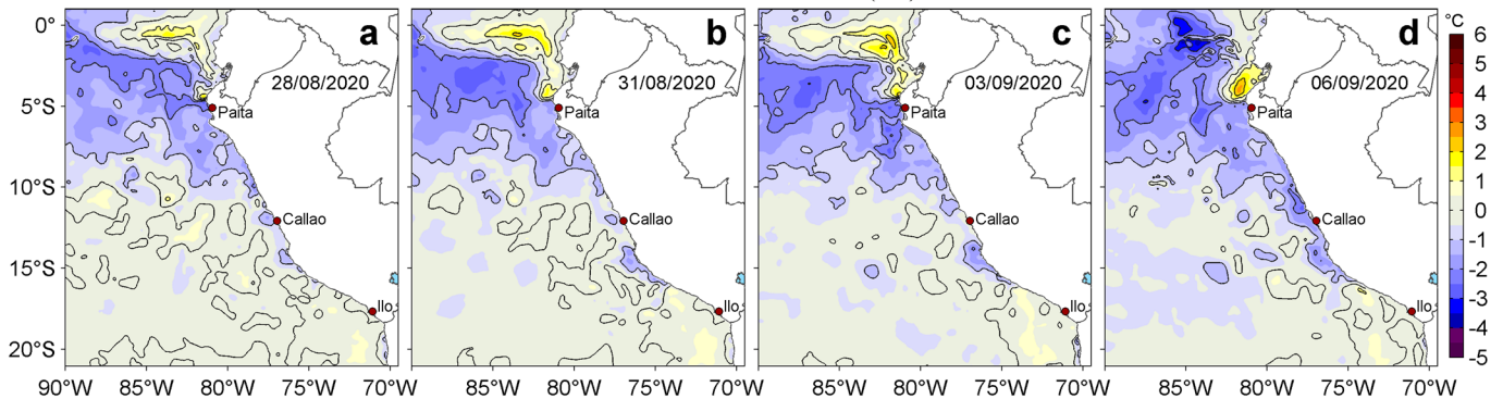
Figura 3. Anomalías de la temperatura superficial del mar (TSM, °C) para los días: a) 28 y b) 31 de agosto, c) 03 y d) 06 de setiembre de 2020. Las anomalías se calcularon respecto de la climatología para el periodo 2007-2016. Datos: OSTIA-UKMO-L4-GLOB-v2.0 (UK Met Office, 2012; Donlon et al, 2012). Procesamiento: LHFMAFIOF/DGIOCC.
