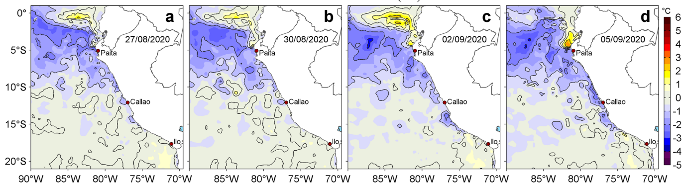
Figura 3. Anomalías de la temperatura superficial del mar (TSM, °C) para los días: a) 27 y b) 30 de agosto, c) 02 y d) 05 de setiembre de 2020. Las anomalías se calcularon respecto de la climatología para el periodo 2007-2016. Datos: OSTIA-UKMO-L4-GLOB-v2.0 (UK Met Office, 2012; Donlon et al, 2012). Procesamiento: LHF/AFIOF/DGIOCC.
