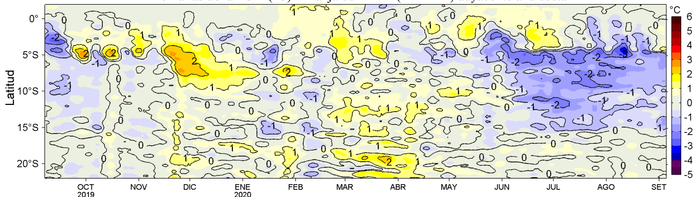
Figura 4. Variación promedio de las anomalías de la temperatura superficial del mar (TSM, °C) para una franja de 60 mn (~111 km) adyacente al litoral peruano para los últimos doce meses al 05 de setiembre de 2020. Datos: OSTIA-UKMO-L4-GLOB-v2.0 (UK Met. Office, 2012; Donlon et al, 2012) disponible en https://podaac.jpl.nasa.gov/dataset/OSTIA-UKMO-L4-GLOB-v2.0 . Las anomalías se calcularon con respecto al periodo 2007-2016. Procesamiento: LHF/AFIOF/DGIOCC.
