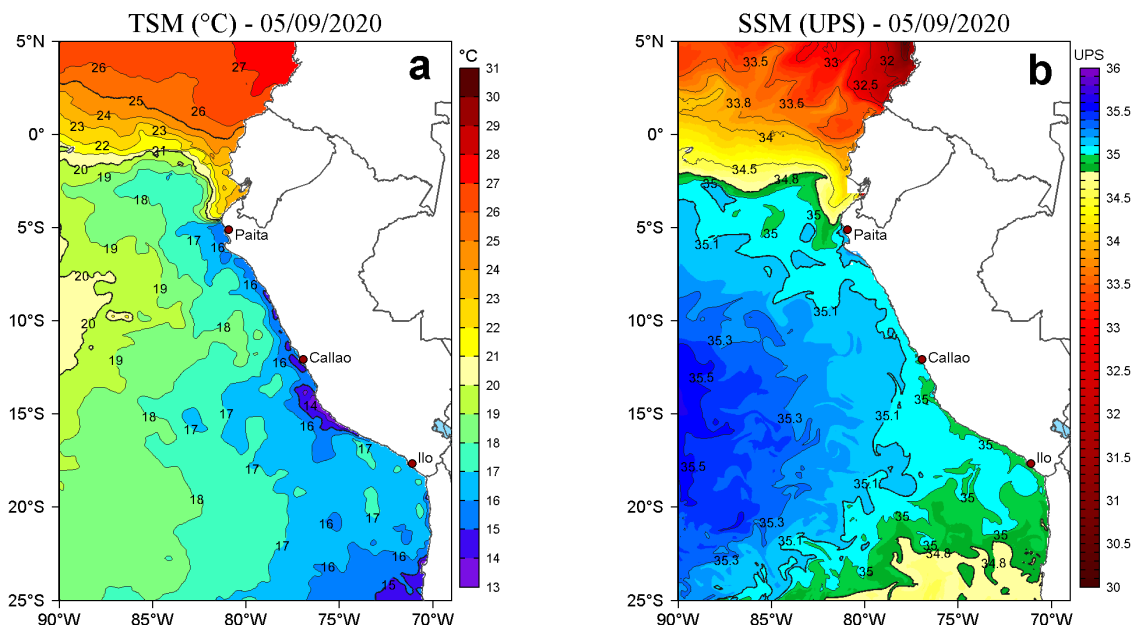
Figura 2. a) Temperatura superficial del mar (TSM, °C) y b) Salinidad superficial del mar (SSM, UPS), para el 05 de setiembre de 2020. Datos: OSTIA-UKMO-L4-GLOB-v2.0 (UK Met Office, 2012; Donlon et al, 2012) disponible en https://podaac.jpl.nasa.gov/dataset/OSTIA-UKMO-L4-GLOB-v2.0 para (a) y Hybrid Coordinate Ocean Model v. GOFS 3.1 (HYCOM; Halliwell et al., 1998; 2000; Bleck, 2001) para (b). Procesamiento: LHF/AFIOF/DGIOCC.
