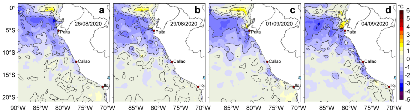
Figura 3. Anomalías de la temperatura superficial del mar (TSM, °C) para los días: a) 26 y b) 29 de agosto, c) 01, d) 04 de setiembre de 2020. Las anomalías se calcularon respecto de la climatología para el periodo 2007-2016. Datos: OSTIA-UKMO-L4-GLOB-v2.0 (UK Met Office, 2012; Donlon et al, 2012). Procesamiento: LHFMA/AFIOF/DGIOCC.
