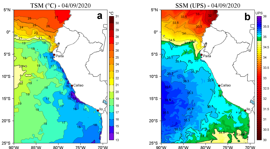
Figura 2. a) Temperatura superficial del mar (TSM, °C) y b) Salinidad superficial del mar (SSM, UPS), para el 04 de setiembre de 2020. Datos: OSTIA-UKMO-L4-GLOB-v2.0 (UK Met Office, 2012; Donlon et al, 2012) disponible en https://podaac.jpl.nasa.gov/dataset/OSTIA-UKMO-L4-GLOB-v2.0 para (a) y Hybrid Coordinate Ocean Model v. GOFS 3.1 (HYCOM; Halliwell et al., 1998; 2000; Bleck, 2001) para (b). Procesamiento: LHFMA/AFIOF/DGIOCC.
