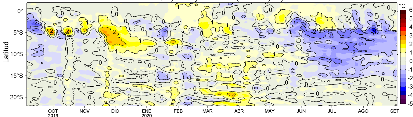
Figura 4. Variación promedio de las anomalías de la temperatura superficial del mar (TSM, °C) para una franja de 60 mn (~111 km) adyacente al litoral peruano para los últimos doce meses al 03 de setiembre de 2020. Datos: OSTIA-UKMO-L4-GLOB-v2.0 (UK Met. Office, 2012; Donlon et al, 2012) disponible en https://podaac.jpl.nasa.gov/dataset/OSTIA-UKMO-L4-GLOB-v2.0 . Las anomalías se calcularon con respecto al periodo 2007-2016. Procesamiento: LHFMA/AFIOF/DGIOCC.
