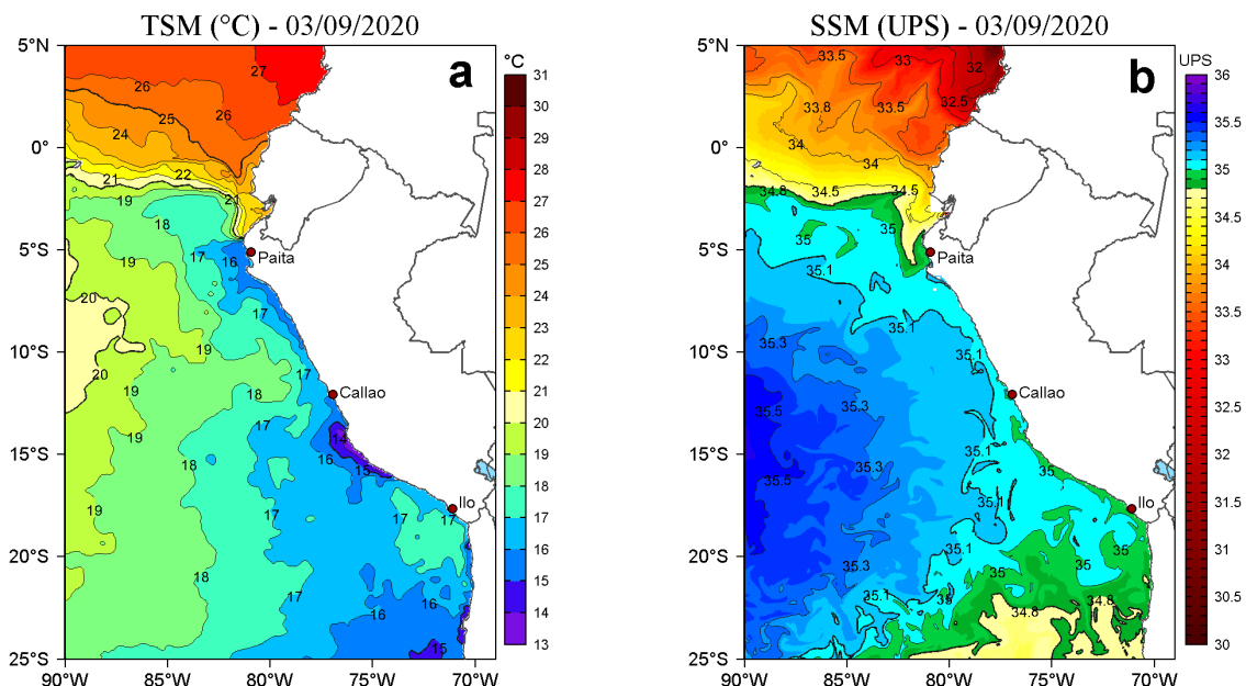
Figura 2. a) Temperatura superficial del mar (TSM, °C) y b) Salinidad superficial del mar (SSM, UPS), para el 03 de setiembre de 2020. Datos: OSTIA-UKMO-L4-GLOB-v2.0 (UK Met Office, 2012; Donlon et al, 2012) disponible en https://podaac.jpl.nasa.gov/dataset/OSTIA-UKMO-L4-GLOB-v2.0 para (a) y Hybrid Coordinate Ocean Model v. GOFS 3.1 (HYCOM; Halliwell et al., 1998; 2000; Bleck, 2001) para (b). Procesamiento: LHFMA/AFIOF/DGIOCC.
