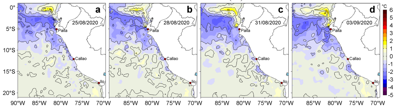
Figura 3. Anomalías de la temperatura superficial del mar (TSM, °C) para los días: a) 25, b) 28 y c) 31 de agosto, d) 03 de setiembre de 2020. Las anomalías se calcularon respecto de la climatología para el periodo 2007-2016. Datos: OSTIA-UKMO-L4-GLOB-v2.0 (UK Met Office, 2012; Donlon et al, 2012). Procesamiento: LHFMA/AFIOF/DGIOCC.
