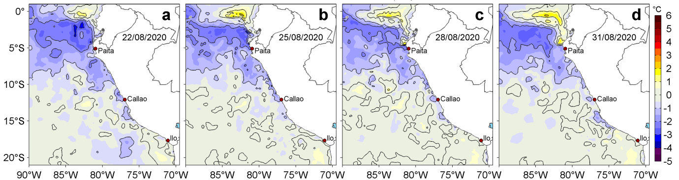
Figura 3. Anomalías de la temperatura superficial del mar (TSM, °C) para los días: a) 22, b) 25, c) 28 y d) 31 de agosto de 2020. Las anomalías se calcularon respecto de la climatología para el periodo 2007-2016. Datos: OSTIA-UKMO-L4-GLOB-v2.0 (UK Met Office, 2012; Donlon et al, 2012). Procesamiento: LHF/AFIOF/DGIOCC.
