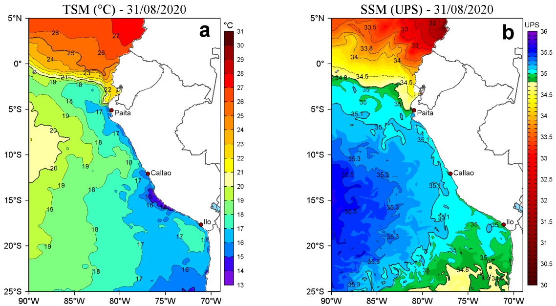
Figura 2. a) Temperatura superficial del mar (TSM, °C) y b) Salinidad superficial del mar (SSM, UPS), para el 31 de agosto de 2020. Datos: OSTIA-UKMO-L4-GLOB-v2.0 (UK Met Office, 2012; Donlon et al, 2012) disponible en https://podaac.jpl.nasa.gov/dataset/OSTIA-UKMO-L4-GLOB-v2.0 para (a) y Hybrid Coordinate Ocean Model v. GOF3 3.1 (HYCOM; Halliwell et al., 1998; 2000; Bleck, 2001) para (b). Procesamiento: LHF/AFIOF/DGIOCC.
