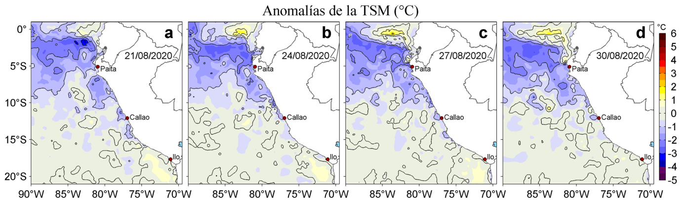
Figura 3. Anomalías de la temperatura superficial del mar (TSM, °C) para los días: a) 21, b) 24, c) 27 y d) 30 de agosto de 2020. Las anomalías se calcularon respecto de la climatología para el periodo 2007-2016. Datos: OSTIA-UKMO-L4-GLOB-v2.0 (UK Met Office, 2012; Donlon et al, 2012). Procesamiento: LHFM/AFIOF/DGIOCC.
