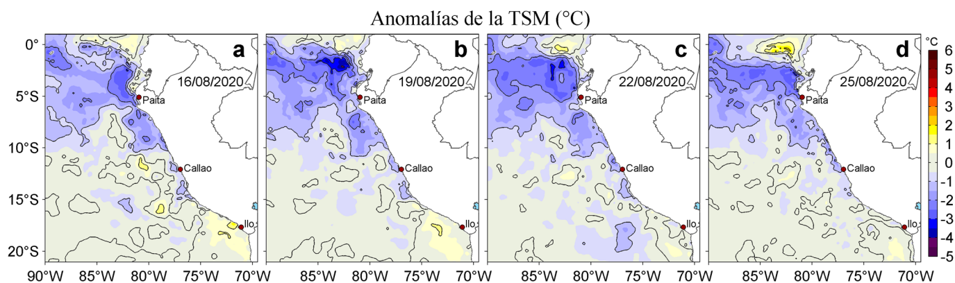
Figura 3. Anomalías de la temperatura superficial del mar (TSM, °C) para los días: a) 16, b) 19, c) 22 y d) 25 de agosto de 2020. Las anomalías se calcularon respecto de la climatología para el periodo 2007-2016. Datos: OSTIA-UKMO-L4-GLOB-v2.0 (UK Met Office, 2012; Donlon et al, 2012). Procesamiento: LHF/AFIOF/DGIOCC.
