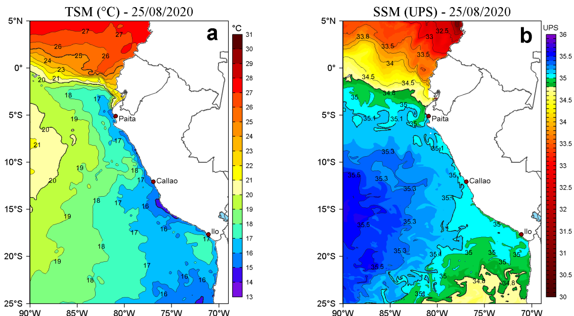
Figura 2. a) Temperatura superficial del mar (TSM, °C) y b) Salinidad superficial del mar (SSM, UPS), para el 25 de agosto de 2020. Datos: OSTIA-UKMO-L4-GLOB-v2.0 (UK Met Office, 2012; Donlon et al, 2012) disponible en https://podaac.jpl.nasa.gov/dataset/OSTIA-UKMO-L4-GLOB-v2.0 para (a) y Hybrid Coordinate Ocean Model v. GOFS 3.1 (HYCOM; Halliwell et al., 1998; 2000; Bleck, 2001) para (b). Procesamiento: LHF/AFIOF/DGIOCC.
