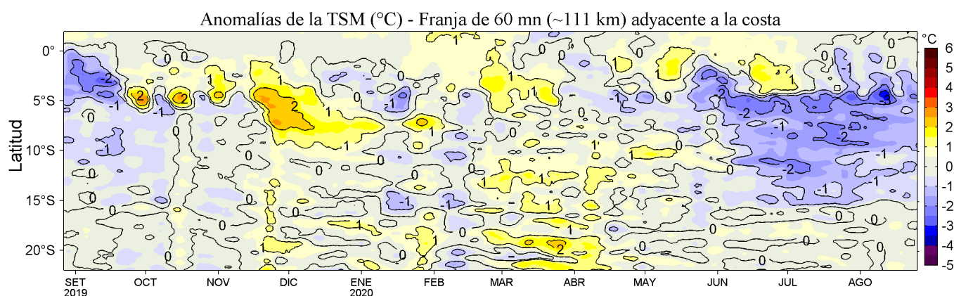
Figura 4. Variación promedio de las anomalías de la temperatura superficial del mar (TSM, °C) para una franja de 60 mn (~111 km) adyacente al litoral peruano para los últimos doce meses al 25 de agosto de 2020. Datos: OSTIA-UKMO-L4-GLOB-v2.0 (UK Met. Office, 2012; Donlon et al, 2012) disponible en https://podaac.jpl.nasa.gov/dataset/OSTIA-UKMO-L4-GLOB-v2.0 . Las anomalías se calcularon con respecto al periodo 2007-2016. Procesamiento: LHF/AFIOF/DGIOCC.
