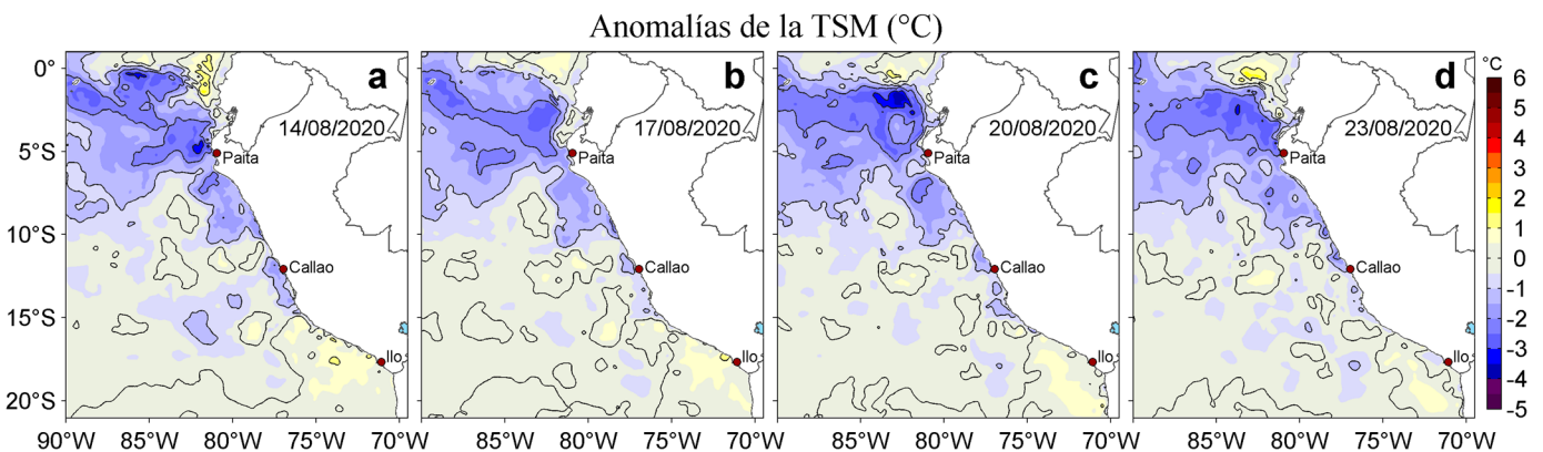
Figura 3. Anomalías de la temperatura superficial del mar (TSM, °C) para los días: a) 14, b) 17, c) 20 y d) 23 de agosto de 2020. Las anomalías se calcularon respecto de la climatología para el periodo 2007-2016. Datos: OSTIA-UKMO-L4-GLOB-v2.0 (UK Met Office, 2012; Donlon et al, 2012). Procesamiento: LHFm/AFIOF/DGIOCC.
