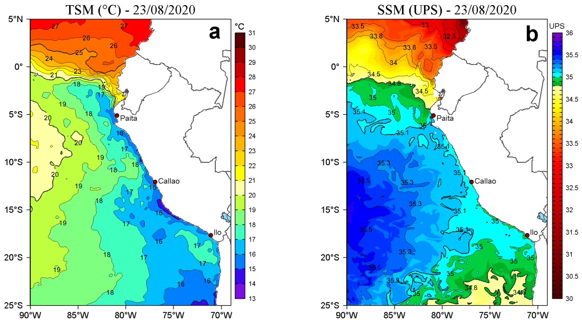
Figura 2. a) Temperatura superficial del mar (TSM, °C) y b) Salinidad superficial del mar (SSM, UPS), para el 23 de agosto de 2020. Datos: OSTIA-UKMO-L4-GLOB-v2.0 (UK Met Office, 2012; Donlon et al, 2012) disponible en https://podaac.jpl.nasa.gov/dataset/OSTIA-UKMO-L4-GLOB-v2.0 para (a) y Hybrid Coordinate Ocean Model v. GOFS 3.1 (HYCOM; Halliwell et al., 1998; 2000; Bleck, 2001) para (b). Procesamiento: LHFm/AFIOF/DGIOCC.
