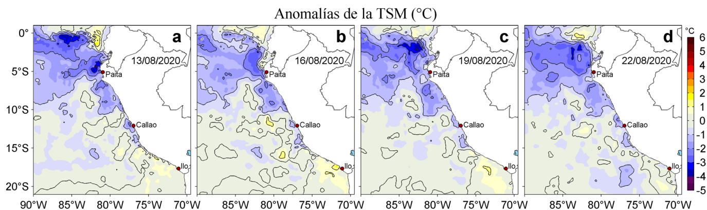
Figura 3. Anomalías de la temperatura superficial del mar (TSM, °C) para los días: a) 13, b) 16, c) 19 y d) 22 de agosto de 2020. Las anomalías se calcularon respecto de la climatología para el periodo 2007-2016. Datos: OSTIA-UKMO-L4-GLOB-v2.0 (UK Met Office, 2012; Donlon et al, 2012). Procesamiento: LHF/AFIOF/DGIOCC.
