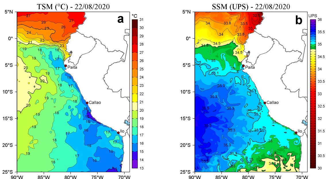
Figura 2. a) Temperatura superficial del mar (TSM, °C) y b) Salinidad superficial del mar (SSM, UPS), para el 22 de agosto de 2020. Datos: OSTIA-UKMO-L4-GLOB-v2.0 (UK Met Office, 2012; Donlon et al, 2012) disponible en https://podaac.jpl.nasa.gov/dataset/OSTIA-UKMO-L4-GLOB-v2.0 para (a) y Hybrid Coordinate Ocean Model v. GOFS 3.1 (HYCOM; Halliwell et al., 1998; 2000; Bleck, 2001) para (b). Procesamiento: LHF/AFIOF/DGIOCC.
