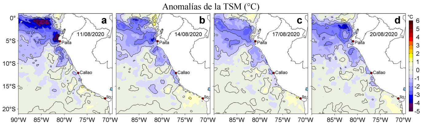
Figura 3. Anomalías de la temperatura superficial del mar (TSM, °C) para los días: a) 11, b) 14, c) 17 y d) 20 de agosto de 2020. Las anomalías se calcularon respecto de la climatología para el periodo 2007-2016. Datos: OSTIA-UKMO-L4-GLOB-v2.0 (UK Met Office, 2012; Donlon et al, 2012). Procesamiento: LHFM/AFIOF/DGIOCC.
