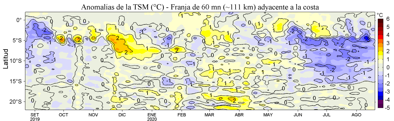
Figura 4. Variación promedio de las anomalías de la temperatura superficial del mar (TSM, °C) para una franja de 60 mn (~111 km) adyacente al litoral peruano para los últimos doce meses al 20 de agosto de 2020. Datos: OSTIA-UKMO-L4-GLOB-v2.0 (UK Met. Office, 2012; Donlon et al, 2012) disponible en https://podaac.jpl.nasa.gov/dataset/OSTIA-UKMO-L4-GLOB-v2.0 . Las anomalías se calcularon con respecto al periodo 2007-2016. Procesamiento: LHFM/AFIOF/DGIOCC.
