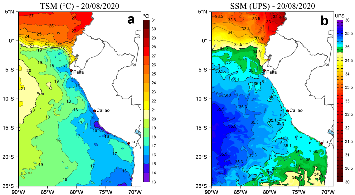
Figura 2. a) Temperatura superficial del mar (TSM, °C) y b) Salinidad superficial del mar (SSM, UPS), para el 20 de agosto de 2020. Datos: OSTIA-UKMO-L4-GLOB-v2.0 (UK Met Office, 2012; Donlon et al, 2012) disponible en https://podaac.jpl.nasa.gov/dataset/OSTIA-UKMO-L4-GLOB-v2.0 para (a) y Hybrid Coordinate Ocean Model v. GOFS 3.1 (HYCOM; Halliwell et al., 1998; 2000; Bleck, 2001) para (b). Procesamiento: LHFM/AFIOF/DGIOCC.
