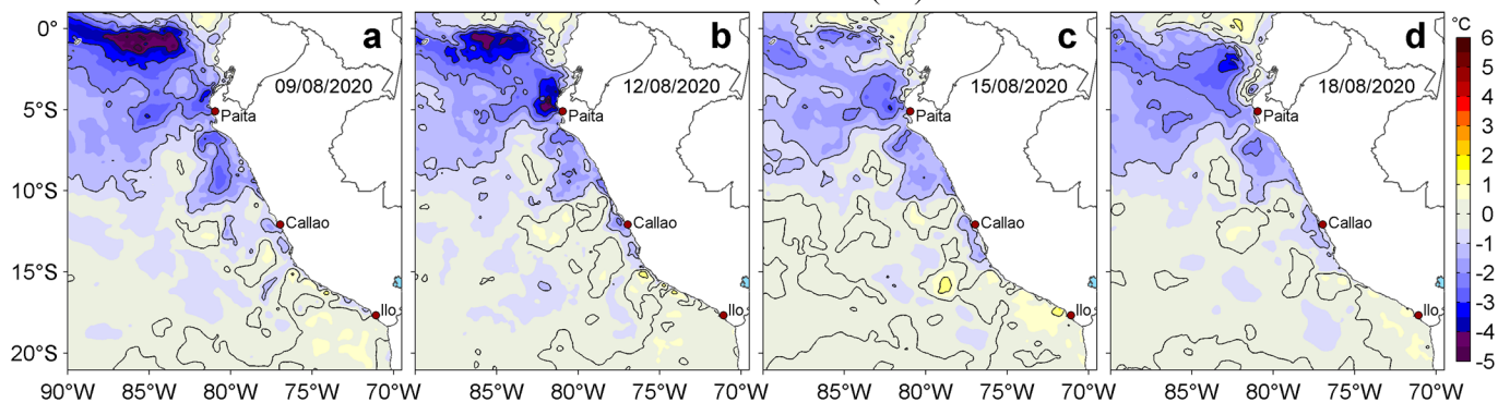
Figura 3. Anomalías de la temperatura superficial del mar (TSM, °C) para los días: a) 09, b) 12, c) 15 y d) 18 de agosto de 2020. Las anomalías se calcularon respecto de la climatología para el periodo 2007-2016. Datos: OSTIA-UKMO-L4-GLOB-v2.0 (UK Met Office, 2012; Donlon et al, 2012). Procesamiento: LHF/AFIOF/DGIOCC.
