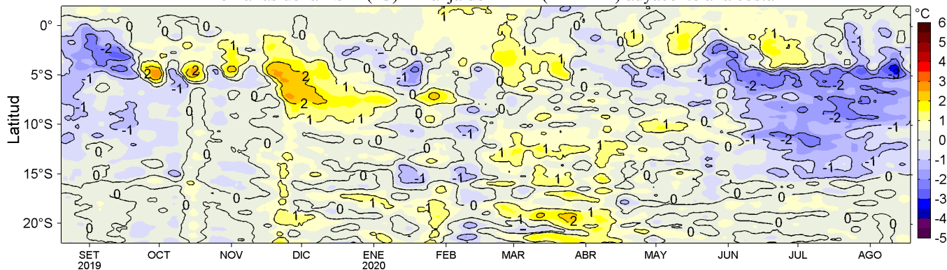
Figura 4. Variación promedio de las anomalías de la temperatura superficial del mar (TSM, °C) para una franja de 60 mn (~111 km) adyacente al litoral peruano para los últimos doce meses al 18 de agosto de 2020. Datos: OSTIA-UKMO-L4-GLOB-v2.0 (UK Met. Office, 2012; Donlon et al, 2012) disponible en https://podaac.jpl.nasa.gov/dataset/OSTIA-UKMO-L4-GLOB-v2.0 . Las anomalías se calcularon con respecto al periodo 2007-2016. Procesamiento: LHF/AFIOF/DGIOCC.
