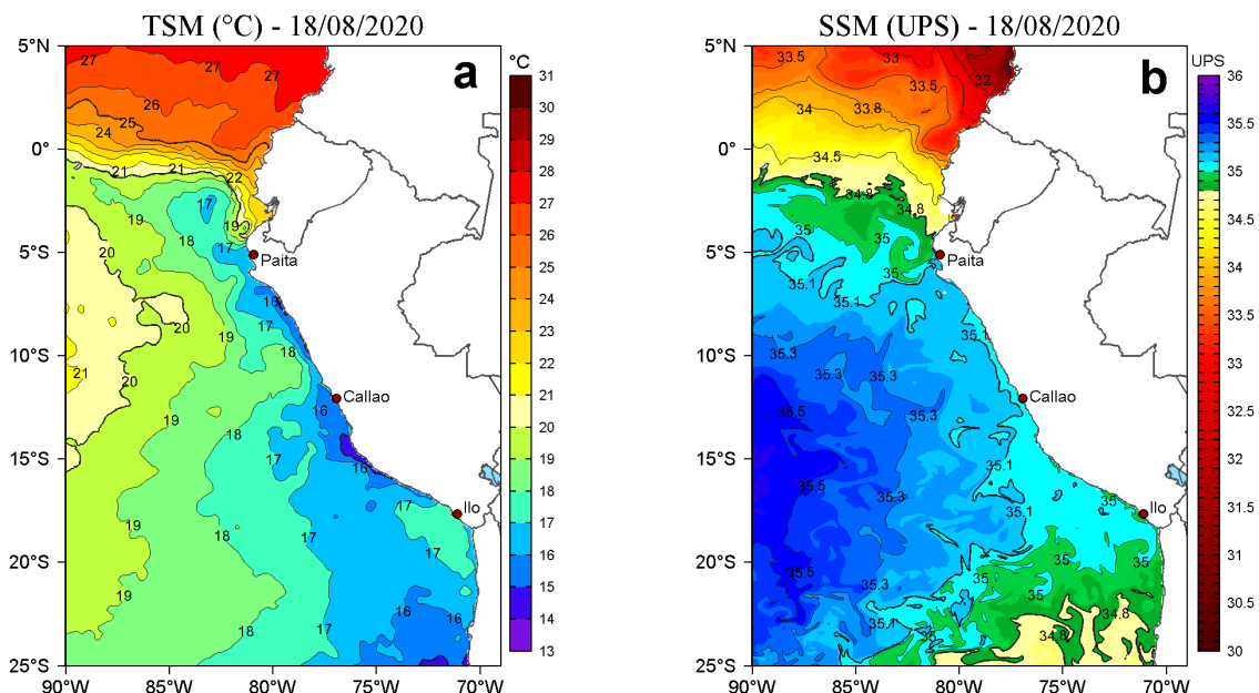
Figura 2. a) Temperatura superficial del mar (TSM, °C) y b) Salinidad superficial del mar (SSM, UPS), para el 18 de agosto de 2020. Datos: OSTIA-UKMO-L4-GLOB-v2.0 (UK Met Office, 2012; Donlon et al, 2012) disponible en https://podaac.jpl.nasa.gov/dataset/OSTIA-UKMO-L4-GLOB-v2.0 para (a) y Hybrid Coordinate Ocean Model v. GOFS 3.1 (HYCOM; Halliwell et al., 1998; 2000; Bleck, 2001) para (b). Procesamiento: LHF/AFIOF/DGIOCC.
