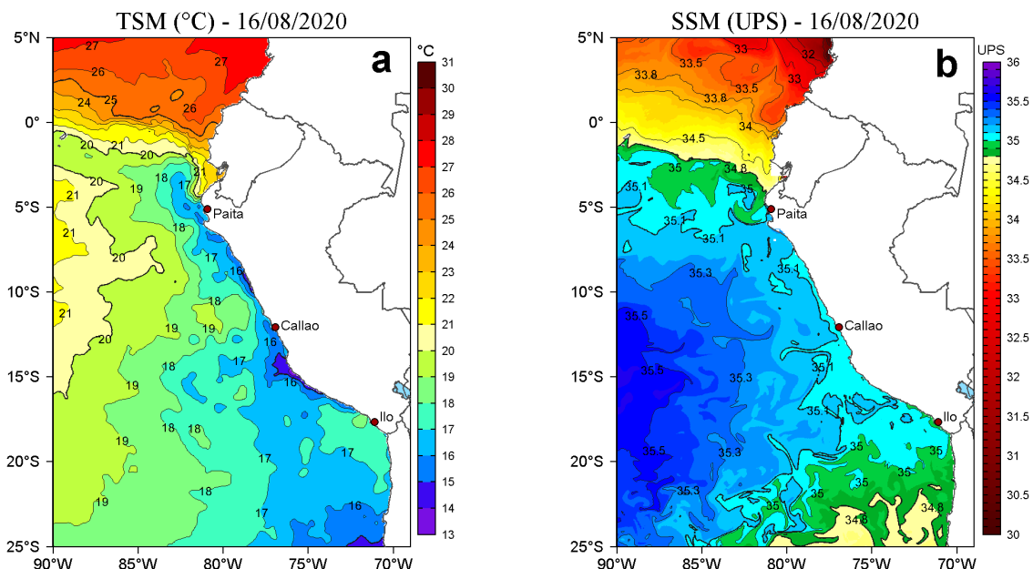
Figura 2. a) Temperatura superficial del mar (TSM, °C) y b) Salinidad superficial del mar (SSM, UPS), para el 16 de agosto de 2020. Datos: OSTIA-UKMO-L4-GLOB-v2.0 (UK Met Office, 2012; Donlon et al, 2012) disponible en https://podaac.jpl.nasa.gov/dataset/OSTIA-UKMO-L4-GLOB-v2.0 para (a) y Hybrid Coordinate Ocean Model v. GOFS 3.1 (HYCOM; Halliwell et al., 1998; 2000; Bleck, 2001) para (b). Procesamiento: LHF/AFIOF/DGIOCC.
