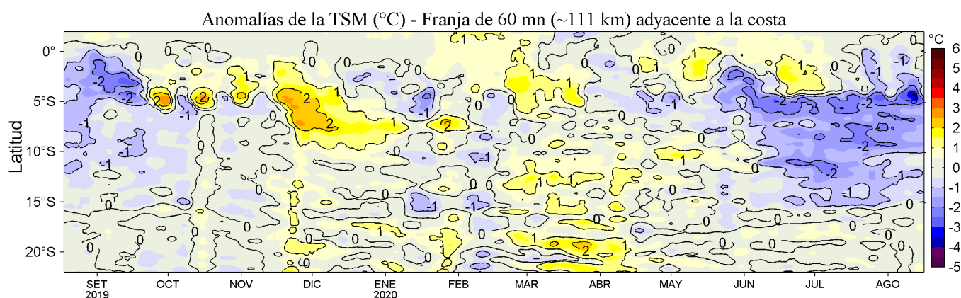
Figura 4. Variación promedio de las anomalías de la temperatura superficial del mar (TSM, °C) para una franja de 60 mn (~111 km) adyacente al litoral peruano para los últimos doce meses al 16 de agosto de 2020. Datos: OSTIA-UKMO-L4-GLOB-v2.0 (UK Met. Office, 2012; Donlon et al, 2012) disponible en https://podaac.jpl.nasa.gov/dataset/OSTIA-UKMO-L4-GLOB-v2.0 . Las anomalías se calcularon con respecto al periodo 2007-2016. Procesamiento: LHF/AFIOF/DGIOCC.
