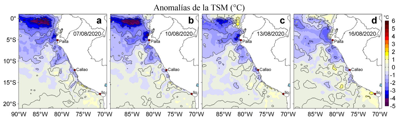
Figura 3. Anomalías de la temperatura superficial del mar (TSM, °C) para los días: a) 07, b) 10, c) 13 y d) 16 de agosto de 2020. Las anomalías se calcularon respecto de la climatología para el periodo 2007-2016. Datos: OSTIA-UKMO-L4-GLOB-v2.0 (UK Met Office, 2012; Donlon et al, 2012). Procesamiento: LHF/AFIOF/DGIOCC.
