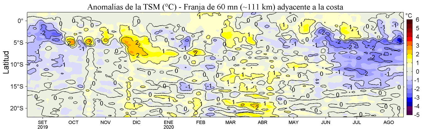
Figura 4. Variación promedio de las anomalías de la temperatura superficial del mar (TSM, °C) para una franja de 60 mn (~111 km) adyacente al litoral peruano para los últimos doce meses al 15 de agosto de 2020. Datos: OSTIA-UKMO-L4-GLOB-v2.0 (UK Met. Office, 2012; Donlon et al, 2012) disponible en https://podaac.jpl.nasa.gov/dataset/OSTIA-UKMO-L4-GLOB-v2.0 . Las anomalías se calcularon con respecto al periodo 2007-2016. Procesamiento: LHF/AFIOF/DGIOCC.
