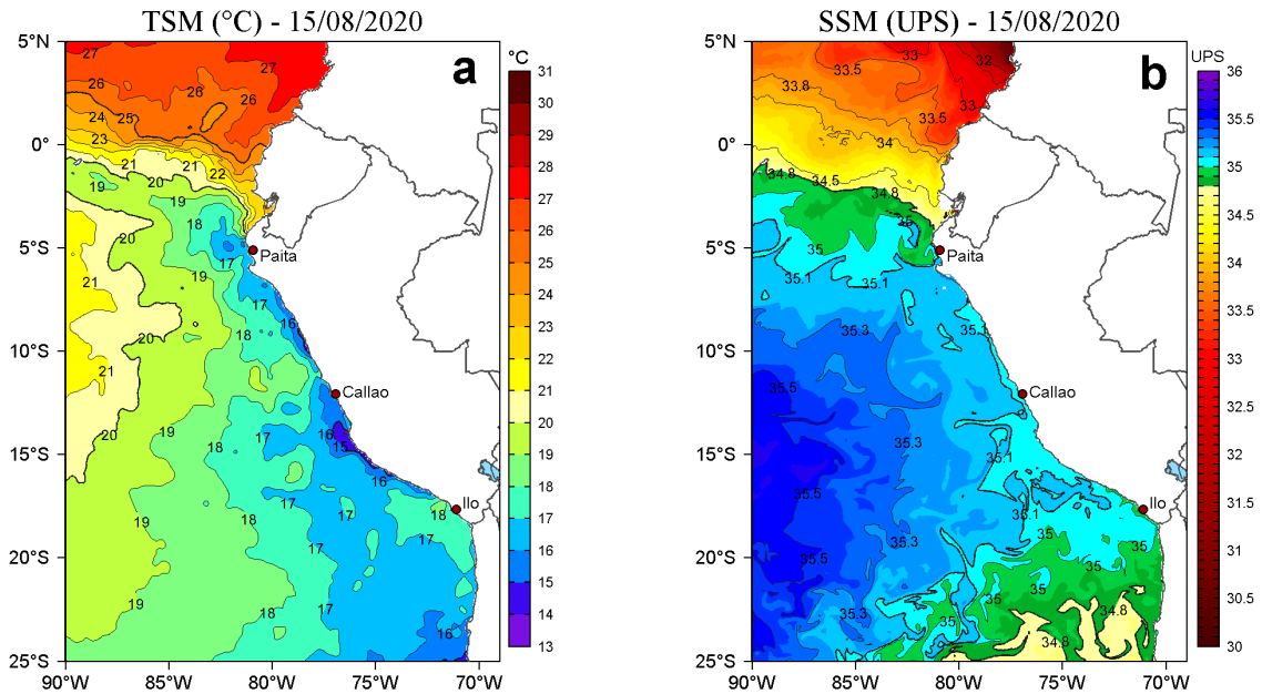
Figura 2. a) Temperatura superficial del mar (TSM, °C) y b) Salinidad superficial del mar (SSM, UPS), para el 15 de agosto de 2020. Datos: OSTIA-UKMO-L4-GLOB-v2.0 (UK Met Office, 2012; Donlon et al, 2012) disponible en https://podaac.jpl.nasa.gov/dataset/OSTIA-UKMO-L4-GLOB-v2.0 para (a) y Hybrid Coordinate Ocean Model v. GOFs 3.1 (HYCOM; Halliwell et al., 1998; 2000; Bleck, 2001) para (b). Procesamiento: LHF/AFIOF/DGIOCC.
