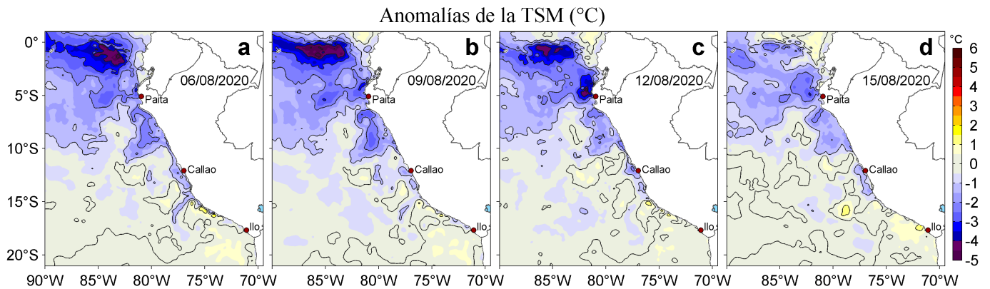
Figura 3. Anomalías de la temperatura superficial del mar (TSM, °C) para los días: a) 06, b) 09, c) 12 y d) 15 de agosto de 2020. Las anomalías se calcularon respecto de la climatología para el periodo 2007-2016. Datos: OSTIA-UKMO-L4-GLOB-v2.0 (UK Met Office, 2012; Donlon et al, 2012). Procesamiento: LHF/AFIOF/DGIOCC.
