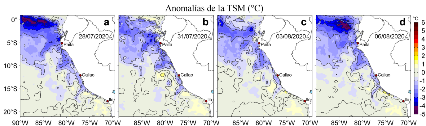
Figura 3. Anomalías de la temperatura superficial del mar (TSM, °C) para los días: a) 28 y b) 31 de julio, c) 03 y d) 06 de agosto de 2020. Las anomalías se calcularon respecto de la climatología para el periodo 2007-2016. Datos: OSTIA-UKMO-L4-GLOB-v2.0 (UK Met Office, 2012; Donlon et al, 2012). Procesamiento: LHF/AFIOF/DGIOCC.
