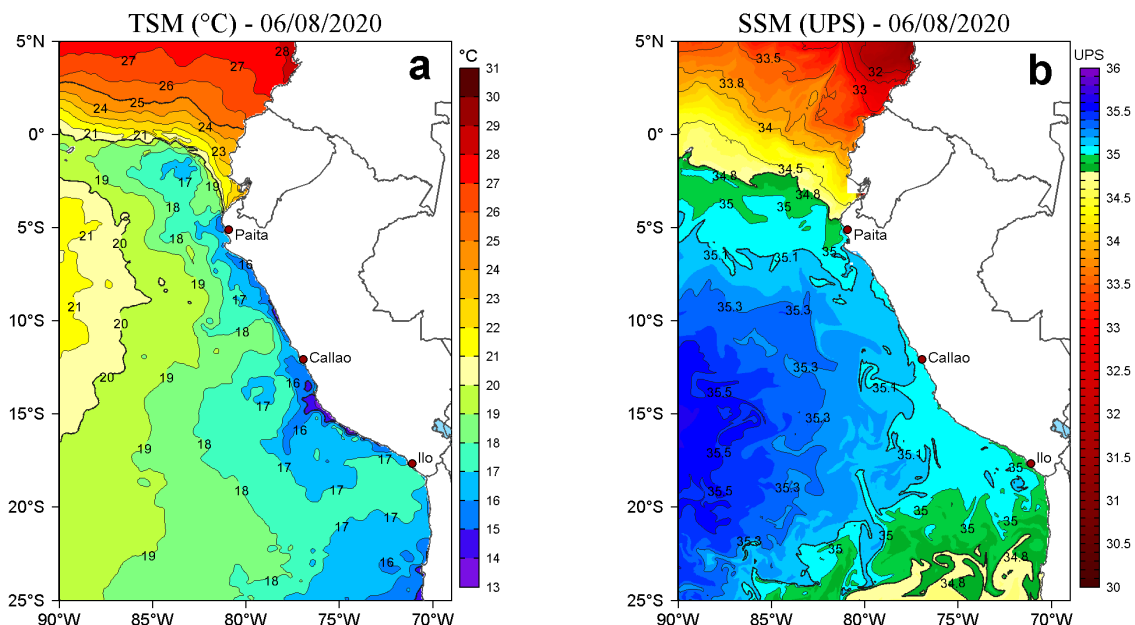
Figura 2. a) Temperatura superficial del mar (TSM, °C) y b) Salinidad superficial del mar (SSM, UPS), para el 06 de agosto de 2020. Datos: OSTIA-UKMO-L4-GLOB-v2.0 (UK Met Office, 2012; Donlon et al, 2012) disponible en https://podaac.jpl.nasa.gov/dataset/OSTIA-UKMO-L4-GLOB-v2.0 para (a) y Hybrid Coordinate Ocean Model v. GOFS 3.1 (HYCOM; Halliwell et al., 1998; 2000; Bleck, 2001) para (b). Procesamiento: LHF/AFIOF/DGIOCC.
