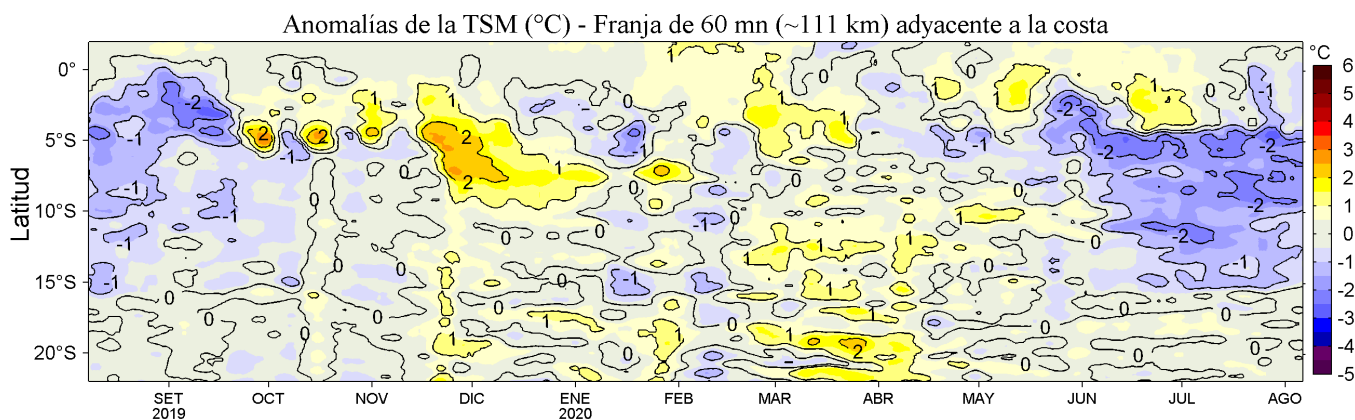
Figura 4. Variación promedio de las anomalías de la temperatura superficial del mar (TSM, °C) para una franja de 60 mn (~111 km) adyacente al litoral peruano para los últimos doce meses al 06 de agosto de 2020. Datos: OSTIA-UKMO-L4-GLOB-v2.0 (UK Met. Office, 2012; Donlon et al, 2012) disponible en https://podaac.jpl.nasa.gov/dataset/OSTIA-UKMO-L4-GLOB-v2.0 . Las anomalías se calcularon con respecto al periodo 2007-2016. Procesamiento: LHF/AFIOF/DGIOCC.
