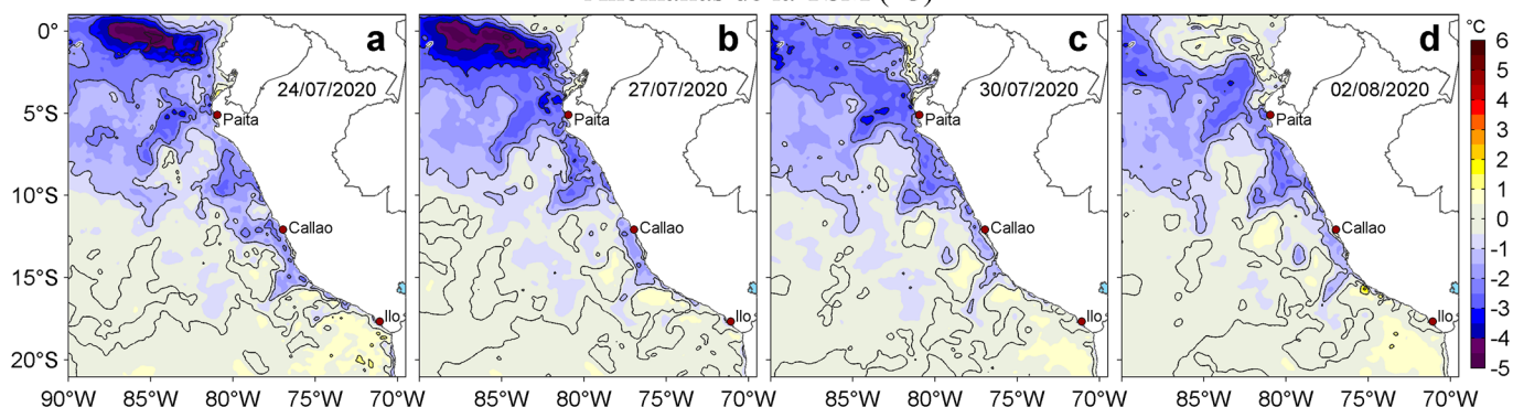
Figura 3. Anomalías de la temperatura superficial del mar (TSM, °C) para los días: a) 24, b) 27 y c) 30 de julio, d) 02 de agosto de 2020. Las anomalías se calcularon respecto de la climatología para el periodo 2007-2016. Datos: OSTIA-UKMO-L4-GLOB-v2.0 (UK Met Office, 2012; Donlon et al, 2012). Procesamiento: LHF/AFIOF/DGIOCC.
