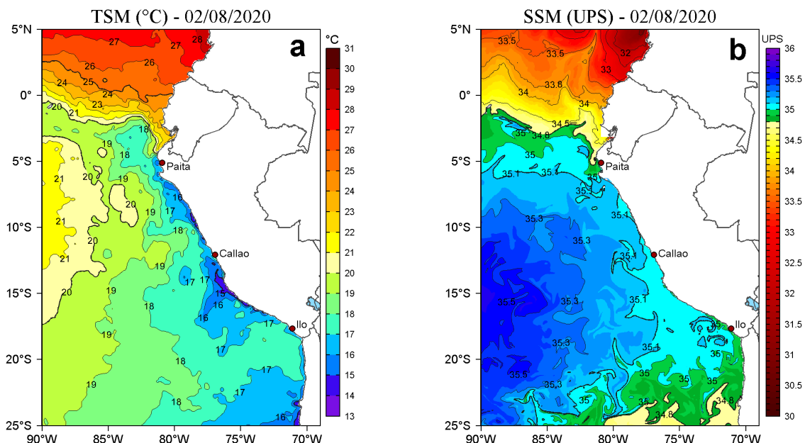
Figura 2. a) Temperatura superficial del mar (TSM, °C) y b) Salinidad superficial del mar (SSM, UPS), para el 02 de agosto de 2020. Datos: OSTIA-UKMO-L4-GLOB-v2.0 (UK Met Office, 2012; Donlon et al, 2012) disponible en https://podaac.jpl.nasa.gov/dataset/OSTIA-UKMO-L4-GLOB-v2.0 para (a) y Hybrid Coordinate Ocean Model v. GOFS 3.1 (HYCOM; Halliwell et al., 1998; 2000; Bleck, 2001) para (b). Procesamiento: LHF/AFIOF/DGIOCC.
