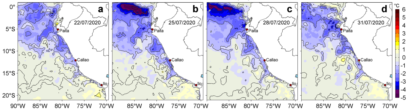
Figura 3. Anomalías de la temperatura superficial del mar (TSM, °C) para los días: a) 22, b) 25, c) 28 y d) 31 de julio de 2020. Las anomalías se calcularon respecto de la climatología para el periodo 2007-2016. Datos: OSTIA-UKMO-L4-GLOB-v2.0 (UK Met Office, 2012; Donlon et al, 2012). Procesamiento: LHF/AFIOF/DGIOCC.
