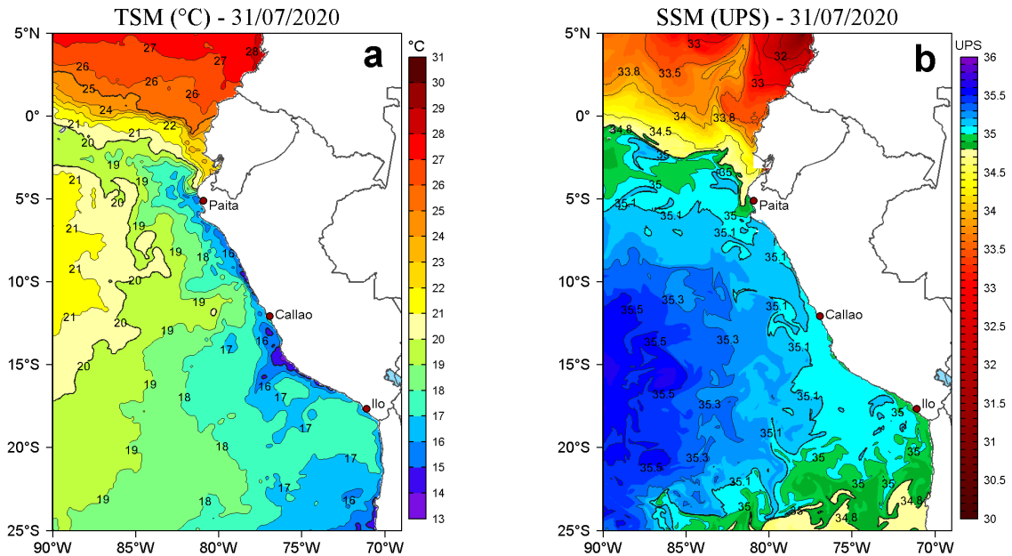
Figura 2. a) Temperatura superficial del mar (TSM, °C) y b) Salinidad superficial del mar (SSM, UPS), para el 31 de julio de 2020. Datos: OSTIA-UKMO-L4-GLOB-v2.0 (UK Met Office, 2012; Donlon et al, 2012) disponible en https://podaac.jpl.nasa.gov/dataset/OSTIA-UKMO-L4-GLOB-v2.0 para (a) y Hybrid Coordinate Ocean Model v. GOFS 3.1 (HYCOM; Halliwell et al., 1998; 2000; Bleck, 2001) para (b). Procesamiento: LHF/AFIOF/DGIOCC.
