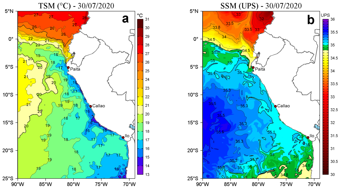
Figura 2. a) Temperatura superficial del mar (TSM, °C) y b) Salinidad superficial del mar (SSM, UPS), para el 30 de julio de 2020. Datos: OSTIA-UKMO-L4-GLOB-v2.0 (UK Met Office, 2012; Donlon et al, 2012) disponible en https://podaac.jpl.nasa.gov/dataset/OSTIA-UKMO-L4-GLOB-v2.0 para (a) y Hybrid Coordinate Ocean Model v. GOFS 3.1 (HYCOM; Halliwell et al., 1998; 2000; Bleck, 2001) para (b). Procesamiento: LHFM/AFIOF/DGIOCC/IMARPE.
