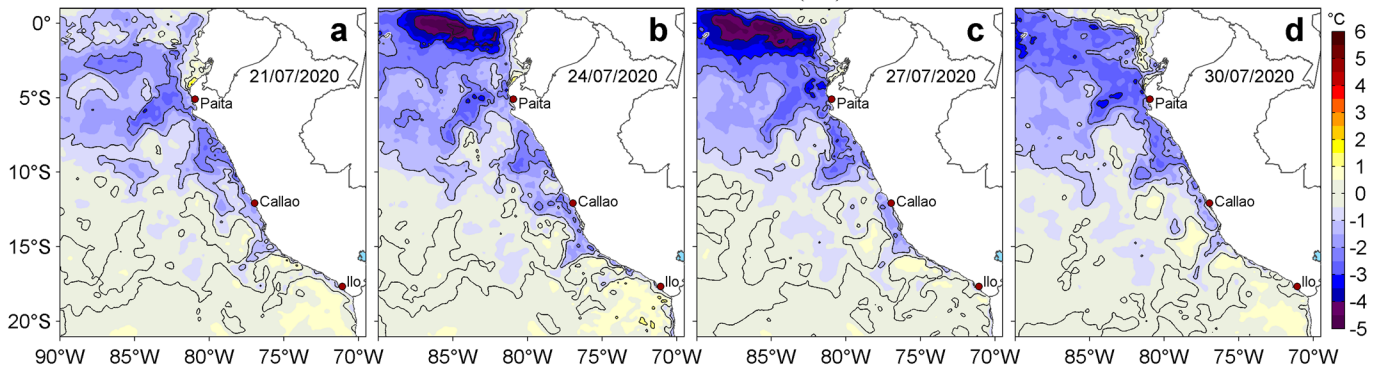
Figura 3. Anomalías de la temperatura superficial del mar (TSM, °C) para los días: a) 21, b) 24, c) 27 y d) 30 de julio de 2020. Las anomalías se calcularon respecto de la climatología para el periodo 2007-2016. Datos: OSTIA-UKMO-L4-GLOB-v2.0 (UK Met Office, 2012; Donlon et al, 2012). Procesamiento: LHFM/AFIOF/DGIOCC/IMARPE.
