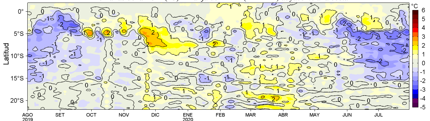
Figura 4. Variación promedio de las anomalías de la temperatura superficial del mar (TSM, °C) para una franja de 60 mn (~111 km) adyacente al litoral peruano para los últimos doce meses al 30 de julio de 2020. Datos: OSTIA-UKMO-L4-GLOB-v2.0 (UK Met. Office, 2012; Donlon et al, 2012) disponible en https://podaac.jpl.nasa.gov/dataset/OSTIA-UKMO-L4-GLOB-v2.0 . Las anomalías se calcularon con respecto al periodo 2007-2016. Procesamiento: LHFM/AFIOF/DGIOCC/IMARPE.
