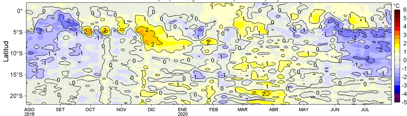
Figura 4. Variación promedio de las anomalías de la temperatura superficial del mar (TSM, °C) para una franja de 60 mn (~111 km) adyacente al litoral peruano para los últimos doce meses al 27 de julio de 2020. Datos: OSTIA-UKMO-L4-GLOB-v2.0 (UK Met. Office, 2012; Donlon et al, 2012) disponible en https://podaac.jpl.nasa.gov/dataset/OSTIA-UKMO-L4-GLOB-v2.0 . Las anomalías se calcularon respecto al periodo 2007-2016. Procesamiento: LHFM/AFIOF/DGIOCC/IMARPE.
