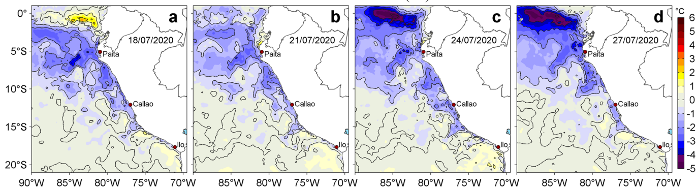
Figura 3. Anomalías de la temperatura superficial del mar (TSM, °C) para los días: a) 18, b) 21, c) 24 y d) 27 de julio de 2020. Las anomalías se calcularon respecto de la climatología para el periodo 2007-2016. Datos: OSTIA-UKMO-L4-GLOB-v2.0 (UK Met Office, 2012; Donlon et al, 2012). Procesamiento: LHFM/AFIOF/DGIOCC/IMARPE.
