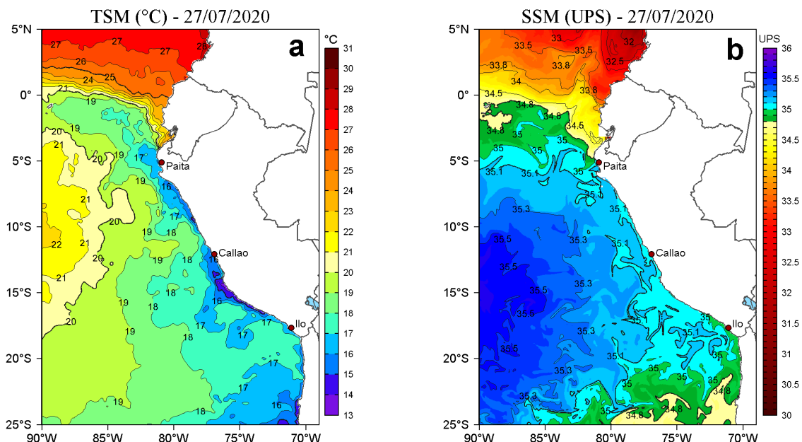
Figura 2. a) Temperatura superficial del mar (TSM, °C) y b) Salinidad superficial del mar (SSM, UPS), para el 27 de julio de 2020. Datos: OSTIA-UKMO-L4-GLOB-v2.0 (UK Met Office, 2012; Donlon et al, 2012) disponible en https://podaac.jpl.nasa.gov/dataset/OSTIA-UKMO-L4-GLOB-v2.0 para (a) y Hybrid Coordinate Ocean Model v. GOFS 3.1 (HYCOM; Halliwell et al., 1998; 2000; Bleck, 2001) para (b). Procesamiento: LHFM/AFIOF/DGIOCC/IMARPE.
