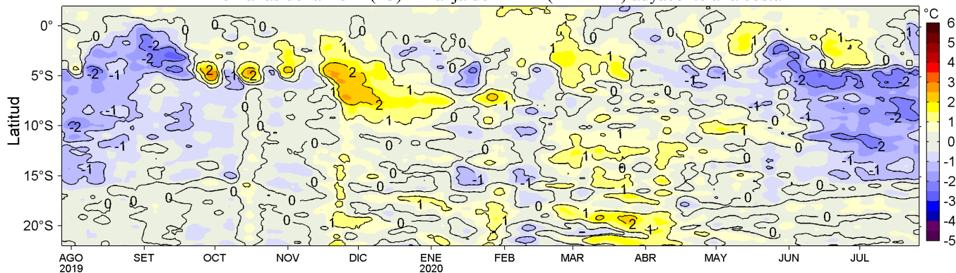
Figura 4. Variación promedio de las anomalías de la temperatura superficial del mar (TSM, °C) para una franja de 60 mn (~111 km) adyacente al litoral peruano para los últimos doce meses al 26 de julio de 2020. Datos: OSTIA-UKMO-L4-GLOB-v2.0 (UK Met. Office, 2012; Donlon et al, 2012) disponible en https://podaac.jpl.nasa.gov/dataset/OSTIA-UKMO-L4-GLOB-v2.0 . Las anomalías se calcularon con respecto al periodo 2007-2016. Procesamiento: LHFm/AFIOF/DGIOCC/IMARPE.
