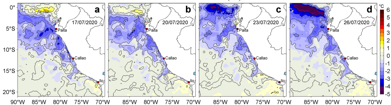
Figura 3. Anomalías de la temperatura superficial del mar (TSM, °C) para los días: a) 17, b) 20, c) 23 y d) 26 de julio de 2020. Las anomalías se calcularon respecto de la climatología para el periodo 2007-2016. Datos: OSTIA-UKMO-L4-GLOB-v2.0 (UK Met Office, 2012; Donlon et al, 2012). Procesamiento: LHFm/AFIOF/DGIOCC/IMARPE.
