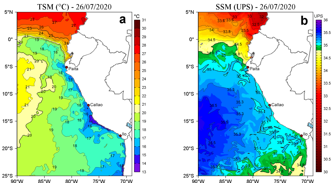
Figura 2. a) Temperatura superficial del mar (TSM, °C) y b) Salinidad superficial del mar (SSM, UPS), para el 26 de julio de 2020. Datos: OSTIA-UKMO-L4-GLOB-v2.0 (UK Met Office, 2012; Donlon et al, 2012) disponible en https://podaac.jpl.nasa.gov/dataset/OSTIA-UKMO-L4-GLOB-v2.0 para (a) y Hybrid Coordinate Ocean Model v. GOFS 3.1 (HYCOM; Halliwell et al., 1998; 2000; Bleck, 2001) para (b). Procesamiento: LHFm/AFIOF/DGIOCC/IMARPE.
