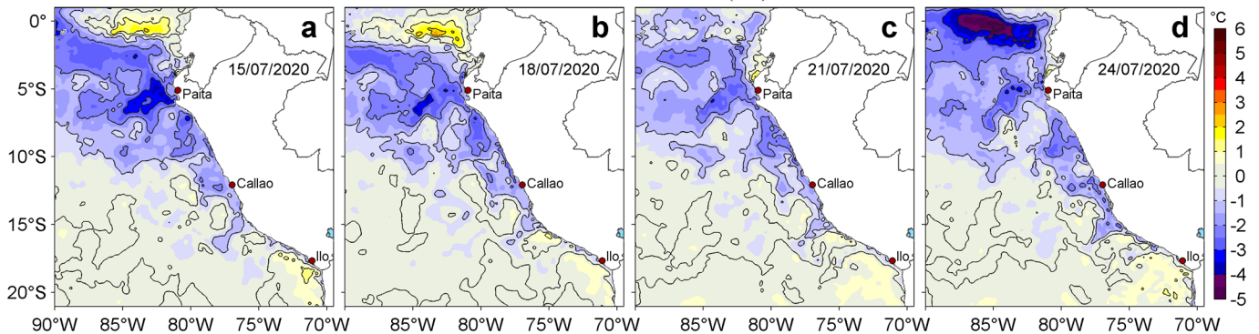
Figura 3. Anomalías de la temperatura superficial del mar (TSM, °C) para los días: a) 15, b) 18, c) 21 y d) 24 de julio de 2020. Las anomalías se calcularon respecto de la climatología para el periodo 2007-2016. Datos: OSTIA-UKMO-L4-GLOB-v2.0 (UK Met Office, 2012; Donlon et al, 2012). Procesamiento: LHF/AFIOF/DGIOCC/IMARPE.
