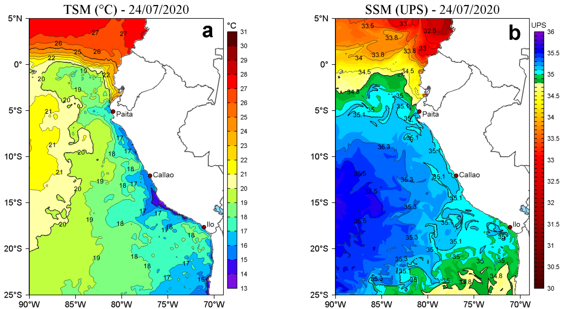
Figura 2. a) Temperatura superficial del mar (TSM, °C) y b) Salinidad superficial del mar (SSM, UPS), para el 24 de julio de 2020. Datos: OSTIA-UKMO-L4-GLOB-v2.0 (UK Met Office, 2012; Donlon et al, 2012) disponible en https://podaac.jpl.nasa.gov/dataset/OSTIA-UKMO-L4-GLOB-v2.0 para (a) y Hybrid Coordinate Ocean Model v. GOFS 3.1 (HYCOM; Halliwell et al., 1998; 2000; Bleck, 2001) para (b). Procesamiento: LHF/AFIOF/DGIOCC/IMARPE.
