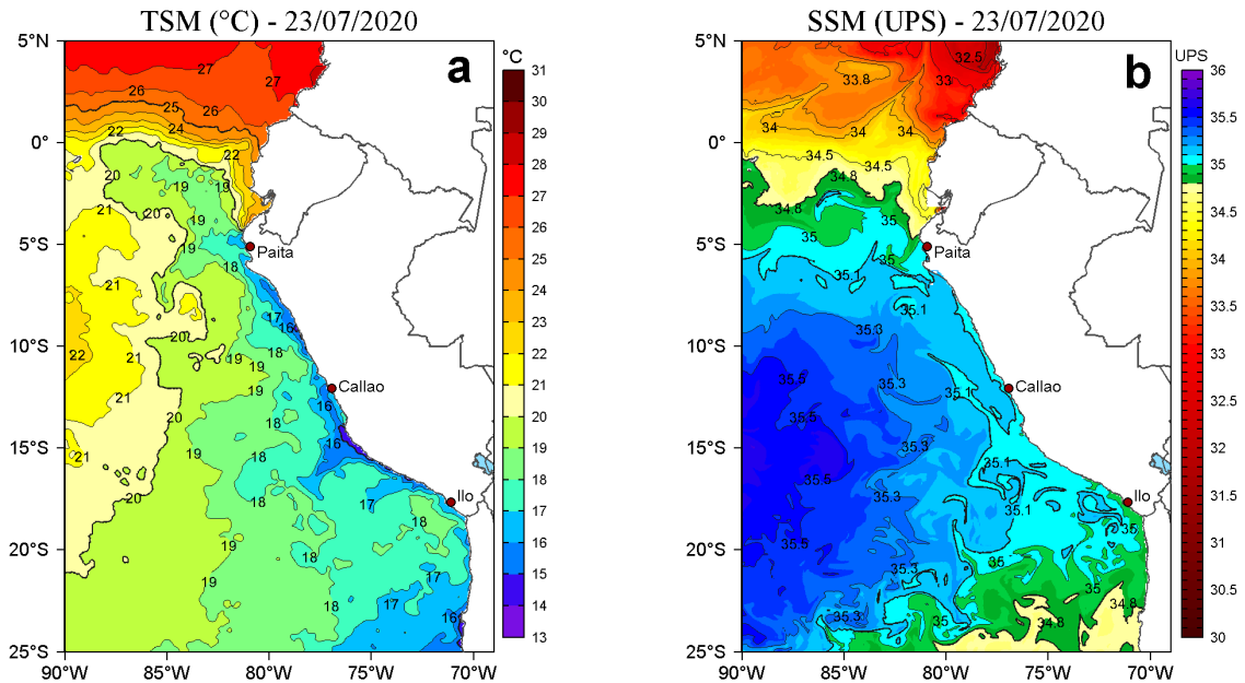
Figura 2. a) Temperatura superficial del mar (TSM, °C) y b) Salinidad superficial del mar (SSM, UPS), para el 23 de julio de 2020. Datos: OSTIA-UKMO-L4-GLOB-v2.0 (UK Met Office, 2012; Donlon et al, 2012) disponible en https://podaac.jpl.nasa.gov/dataset/OSTIA-UKMO-L4-GLOB-v2.0 para (a) y Hybrid Coordinate Ocean Model v. GOFS 3.1 (HYCOM; Halliwell et al., 1998; 2000; Bleck, 2001) para (b). Procesamiento: LHFM/AFIOF/DGIOCC/IMARPE.
