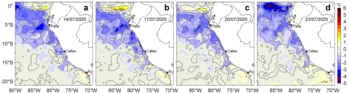
Figura 3. Anomalías de la temperatura superficial del mar (TSM, °C) para los días: a) 14, b) 17, c) 20 y d) 23 de julio de 2020. Las anomalías se calcularon respecto de la climatología para el periodo 2007-2016. Datos: OSTIA-UKMO-L4-GLOB-v2.0 (UK Met Office, 2012; Donlon et al, 2012). Procesamiento: LHFM/AFIOF/DGIOCC/IMARPE.
