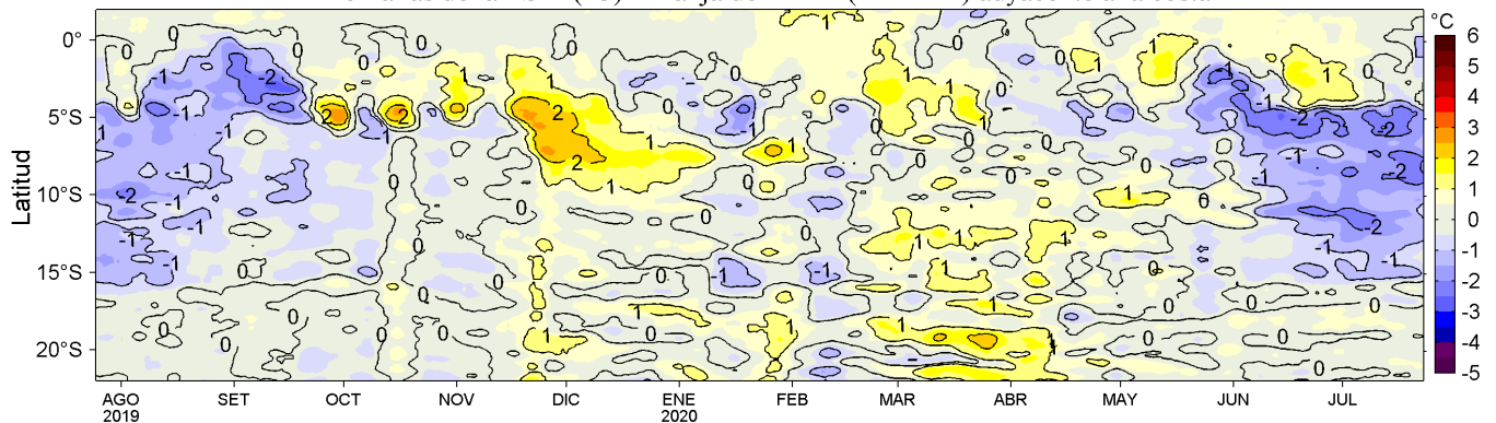
Figura 4. Variación promedio de las anomalías de la temperatura superficial del mar (TSM, °C) para una franja de 60 mn (~111 km) adyacente al litoral peruano para los últimos doce meses al 23 de julio de 2020. Datos: OSTIA-UKMO-L4-GLOB-v2.0 (UK Met. Office, 2012; Donlon et al, 2012) disponible en https://podaac.jpl.nasa.gov/dataset/OSTIA-UKMO-L4-GLOB-v2.0 . Las anomalías se calcularon con respecto al periodo 2007-2016. Procesamiento: LHFM/AFIOF/DGIOCC/IMARPE.
