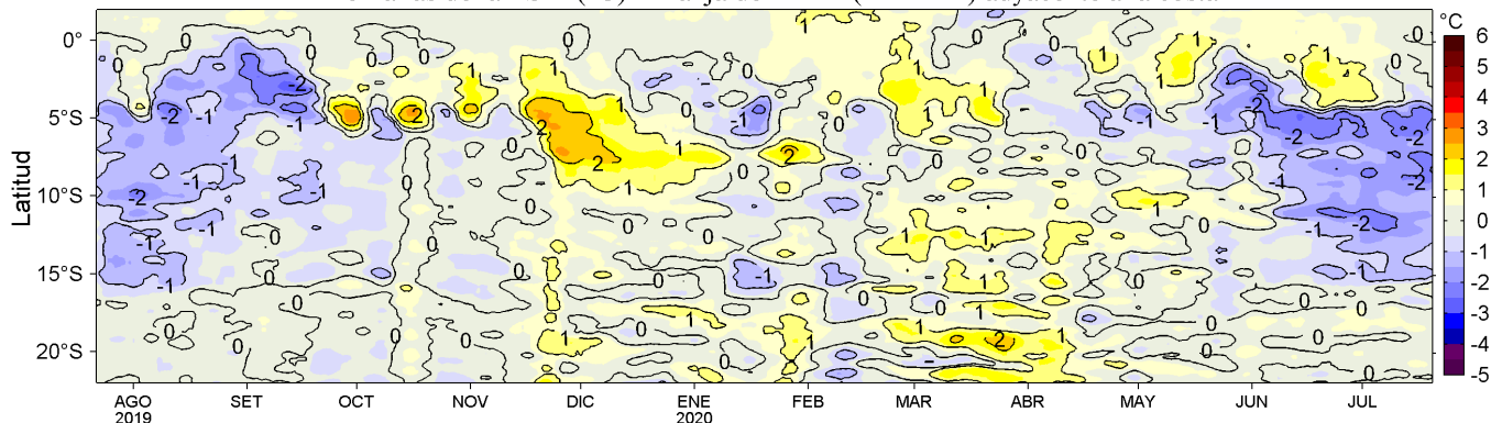
Figura 4. Variación promedio de las anomalías de la temperatura superficial del mar (TSM, °C) para una franja de 60 mn (~111 km) adyacente al litoral peruano para los últimos doce meses al 20 de julio de 2020. Datos: OSTIA-UKMO-L4-GLOB-v2.0 (UK Met. Office, 2012; Donlon et al, 2012) disponible en https://podaac.jpl.nasa.gov/dataset/OSTIA-UKMO-L4-GLOB-v2.0 . Las anomalías se calcularon con respecto al periodo 2007-2016. Procesamiento: LHFM/AFIOF/DGIOCC/IMARPE.
