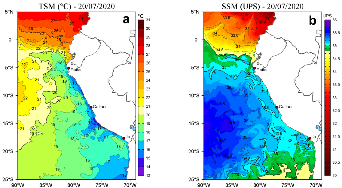
Figura 2. a) Temperatura superficial del mar (TSM, °C) y b) Salinidad superficial del mar (SSM, UPS), para el 20 de julio de 2020. Datos: OSTIA-UKMO-L4-GLOB-v2.0 (UK Met Office, 2012; Donlon et al, 2012) disponible en https://podaac.jpl.nasa.gov/dataset/OSTIA-UKMO-L4-GLOB-v2.0 para (a) y Hybrid Coordinate Ocean Model v. GOFS 3.1 (HYCOM; Halliwell et al., 1998; 2000; Bleck, 2001) para (b). Procesamiento: LHFM/AFIOF/DGIOCC/IMARPE.
