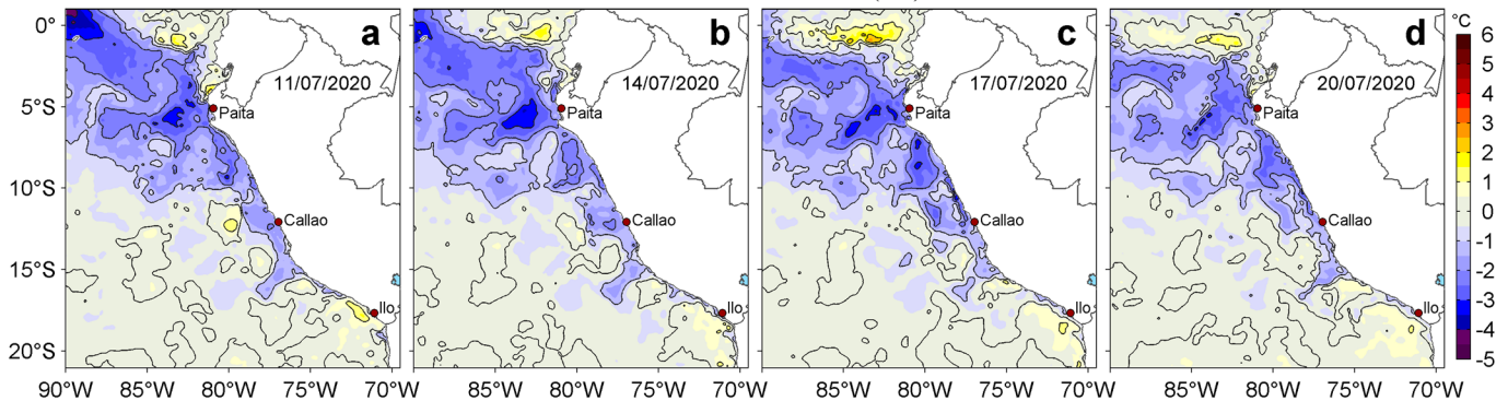
Figura 3. Anomalías de la temperatura superficial del mar (TSM, °C) para los días: a) 11, b) 14, c) 17 y d) 20 de julio de 2020. Las anomalías se calcularon respecto de la climatología para el periodo 2007-2016. Datos: OSTIA-UKMO-L4-GLOB-v2.0 (UK Met Office, 2012; Donlon et al, 2012). Procesamiento: LHFM/AFIOF/DGIOCC/IMARPE.
