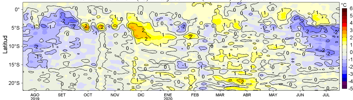
Figura 4. Variación promedio de las anomalías de la temperatura superficial del mar (TSM, °C) para una franja de 60 mn (~111 km) adyacente al litoral peruano para los últimos doce meses al 16 de julio de 2020. Datos: OSTIA-UKMO-L4-GLOB-v2.0 (UK Met. Office, 2012; Donlon et al, 2012) disponible en https://podaac.jpl.nasa.gov/dataset/OSTIA-UKMO-L4-GLOB-v2.0 . Las anomalías se calcularon con respecto al periodo 2007-2016. Procesamiento: LHF/AFIOF/DGIOCC/IMARPE.
