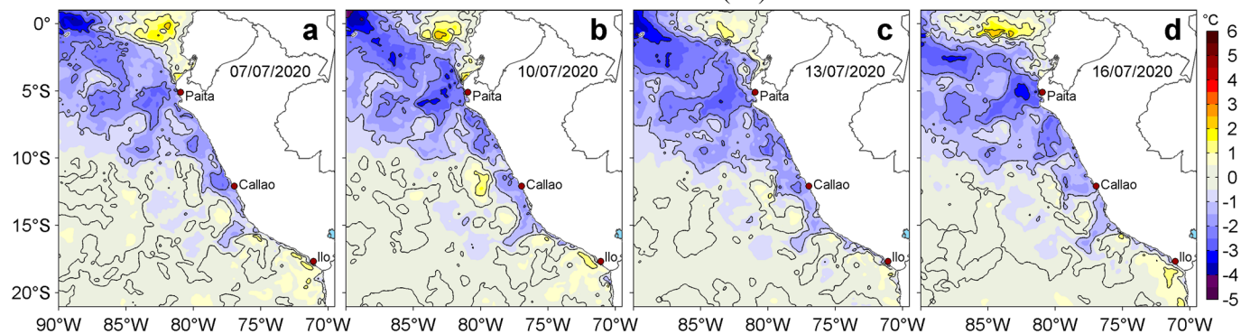
Figura 3. Anomalías de la temperatura superficial del mar (TSM, °C) para los días: a) 07, b) 10, c) 13 y d) 16 de julio de 2020. Las anomalías se calcularon respecto de la climatología para el periodo 2007-2016. Datos: OSTIA-UKMO-L4-GLOB-v2.0 (UK Met Office, 2012; Donlon et al, 2012). Procesamiento: LHF/AFIOF/DGIOCC/IMARPE.
