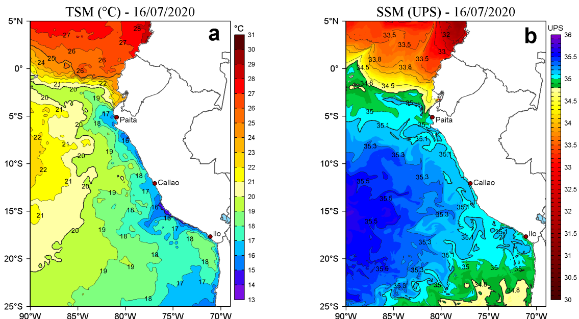
Figura 2. a) Temperatura superficial del mar (TSM, °C) y b) Salinidad superficial del mar (SSM, UPS), para el 16 de julio de 2020. Datos: OSTIA-UKMO-L4-GLOB-v2.0 (UK Met Office, 2012; Donlon et al, 2012) disponible en https://podaac.jpl.nasa.gov/dataset/OSTIA-UKMO-L4-GLOB-v2.0 para (a) y Hybrid Coordinate Ocean Model v. GOFS 3.1 (HYCOM; Halliwell et al., 1998; 2000; Bleck, 2001) para (b). Procesamiento: LHF/AFIOF/DGIOCC/IMARPE.
