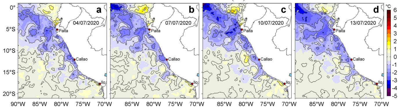
Figura 3. Anomalías de la temperatura superficial del mar (TSM, °C) para los días: a) 04, b) 07, c) 10 y d) 13 de julio de 2020. Las anomalías se calcularon respecto de la climatología para el periodo 2007-2016. Datos: OSTIA-UKMO-L4-GLOB-v2.0 (UK Met Office, 2012; Donlon et al, 2012). Procesamiento: LHF/M/AFIOF/DGIOCC/IMARPE.
