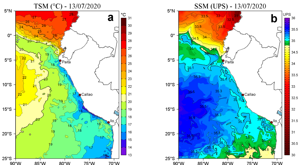
Figura 2. a) Temperatura superficial del mar (TSM, °C) y b) Salinidad superficial del mar (SSM, UPS), para el 13 de julio de 2020. Datos: OSTIA-UKMO-L4-GLOB-v2.0 (UK Met Office, 2012; Donlon et al, 2012) disponible en https://podaac.jpl.nasa.gov/dataset/OSTIA-UKMO-L4-GLOB-v2.0 para (a) y Hybrid Coordinate Ocean Model v. GOFS 3.1 (HYCOM; Halliwell et al., 1998; 2000; Bleck, 2001) para (b). Procesamiento: LHF/M/AFIOF/DGIOCC/IMARPE.
