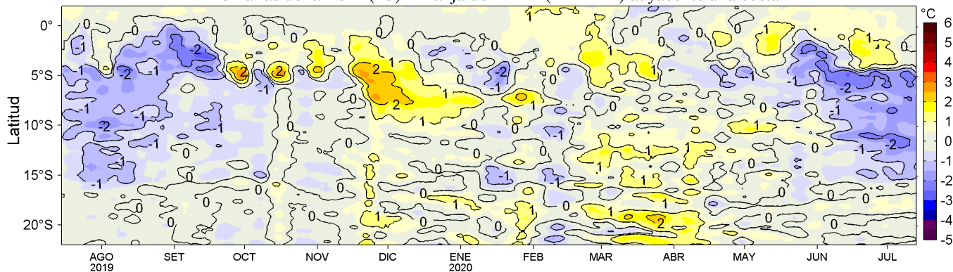
Figura 4. Variación promedio de las anomalías de la temperatura superficial del mar (TSM, °C) para una franja de 60 mn (~111 km) adyacente al litoral peruano para los últimos doce meses al 13 de julio de 2020. Datos: OSTIA-UKMO-L4-GLOB-v2.0 (UK Met. Office, 2012; Donlon et al, 2012) disponible en https://podaac.jpl.nasa.gov/dataset/OSTIA-UKMO-L4-GLOB-v2.0 . Las anomalías se calcularon con respecto al periodo 2007-2016. Procesamiento: LHF/M/AFIOF/DGIOCC/IMARPE.
