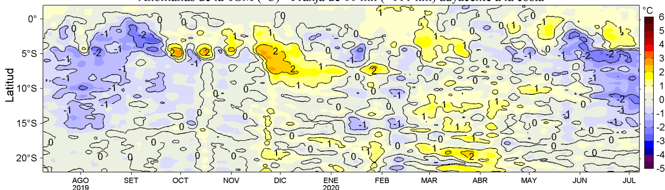
Figura 4. Variación promedio de las anomalías de la temperatura superficial del mar (TSM, °C) para una franja de 60 mn (~111 km) adyacente al litoral peruano para los últimos doce meses al 07 de julio de 2020. Datos: OSTIA-UKMO-L4-GLOB-v2.0 (UK Met. Office, 2012; Donlon et al, 2012) disponible en https://podaac.jpl.nasa.gov/dataset/OSTIA-UKMO-L4-GLOB-v2.0 . Las anomalías se calcularon con respecto al periodo 2007-2016. Procesamiento: LHFm/AFIOF/DGIOCC/IMARPE.
