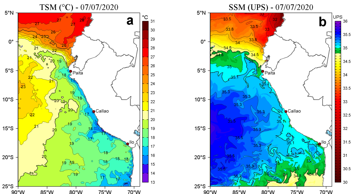
Figura 2. a) Temperatura superficial del mar (TSM, °C) y b) Salinidad superficial del mar (SSM, UPS), para el 07 de julio de 2020. Datos: OSTIA-UKMO-L4-GLOB-v2.0 (UK Met Office, 2012; Donlon et al, 2012) disponible en https://podaac.jpl.nasa.gov/dataset/OSTIA-UKMO-L4-GLOB-v2.0 para (a) y Hybrid Coordinate Ocean Model v. GOFS 3.1 (HYCOM; Halliwell et al., 1998; 2000; Bleck, 2001) para (b). Procesamiento: LHFm/AFIOF/DGIOCC/IMARPE.
