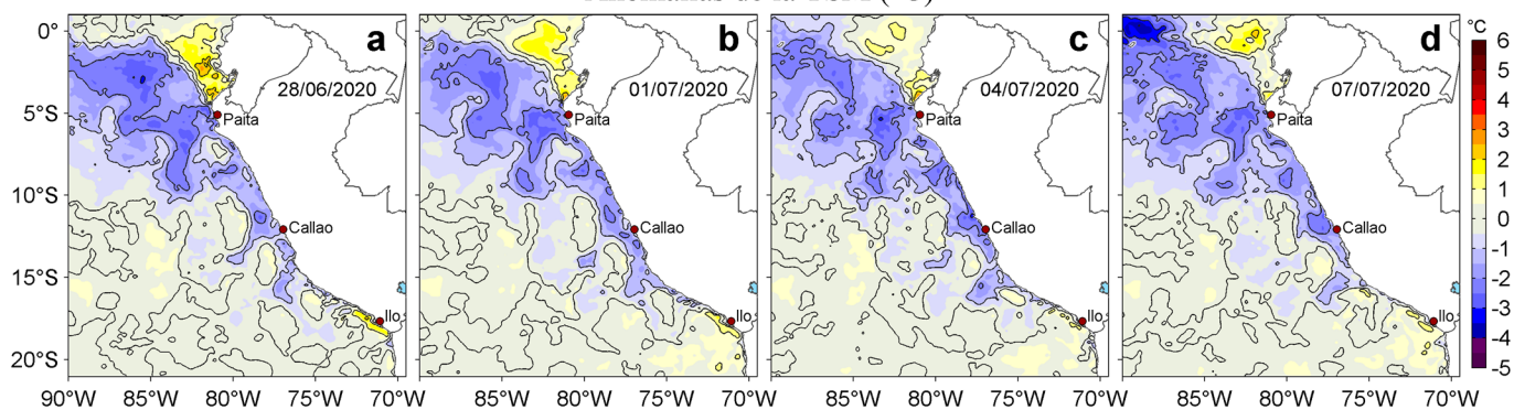
Figura 3. Anomalías de la temperatura superficial del mar (TSM, °C) para los días: a) 28 de junio, b) 01, c) 04 y d) 07 de julio de 2020. Las anomalías se calcularon respecto de la climatología para el periodo 2007-2016. Datos: OSTIA-UKMO-L4-GLOB-v2.0 (UK Met Office, 2012; Donlon et al, 2012). Procesamiento: LHFm/AFIOF/DGIOCC/IMARPE.
