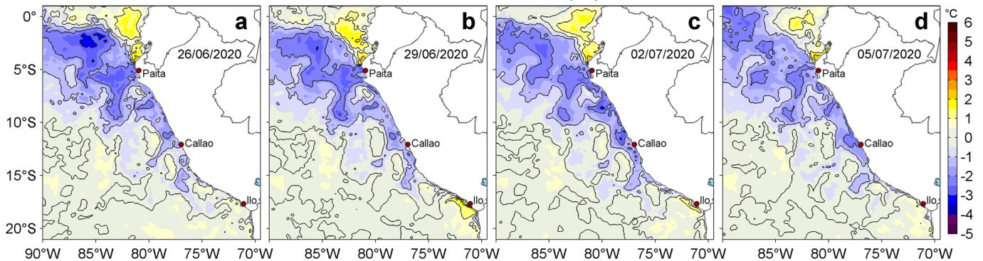
Figura 3. Anomalías de la temperatura superficial del mar (TSM, °C) para los días: a) 26 y b) 29 de junio, c) 02 y d) 05 de julio de 2020. Las anomalías se calcularon respecto de la climatología para el periodo 2007-2016. Datos: OSTIA-UKMO-L4-GLOB-v2.0 (UK Met Office, 2012; Donlon et al, 2012). Procesamiento: LHF/AFIOF/DGIOCC/IMARPE.
