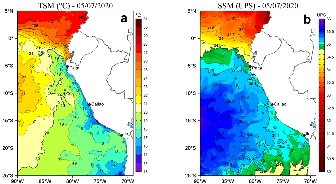
Figura 2. a) Temperatura superficial del mar (TSM, °C) y b) Salinidad superficial del mar (SSM, UPS), para el 05 de julio de 2020. Datos: OSTIA-UKMO-L4-GLOB-v2.0 (UK Met Office, 2012; Donlon et al, 2012) disponible en https://podaac.jpl.nasa.gov/dataset/OSTIA-UKMO-L4-GLOB-v2.0 para (a) y Hybrid Coordinate Ocean Model v. GOFS 3.1 (HYCOM; Halliwell et al., 1998; 2000; Bleck, 2001) para (b). Procesamiento: LHF/AFIOF/DGIOCC/IMARPE.
