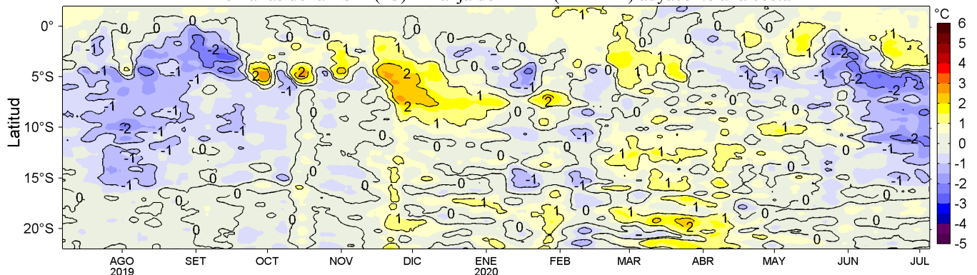
Figura 4. Variación promedio de las anomalías de la temperatura superficial del mar (TSM, °C) para una franja de 60 mn (~111 km) adyacente al litoral peruano para los últimos doce meses al 05 de julio de 2020. Datos: OSTIA-UKMO-L4-GLOB-v2.0 (UK Met. Office, 2012; Donlon et al, 2012) disponible en https://podaac.jpl.nasa.gov/dataset/OSTIA-UKMO-L4-GLOB-v2.0 . Las anomalías se calcularon con respecto al periodo 2007-2016. Procesamiento: LHF/AFIOF/DGIOCC/IMARPE.
