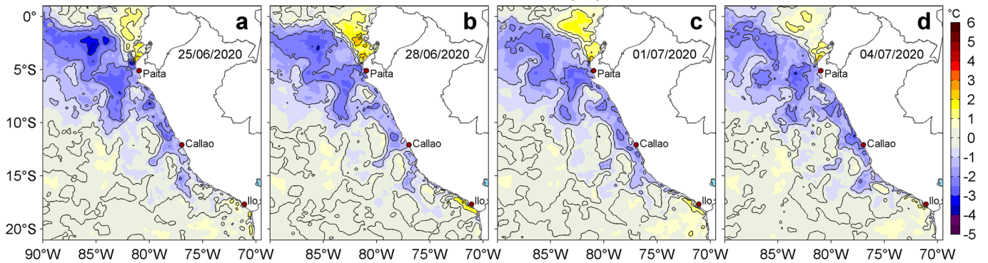
Figura 3. Anomalías de la temperatura superficial del mar (TSM, °C) para los días: a) 25 y b) 28 de junio, c) 01 y d) 04 de julio de 2020. Las anomalías se calcularon respecto de la climatología para el periodo 2007-2016. Datos: OSTIA-UKMO-L4-GLOB-v2.0 (UK Met Office, 2012; Donlon et al, 2012). Procesamiento: LHF/AFIOF/DGIOCC/IMARPE.
