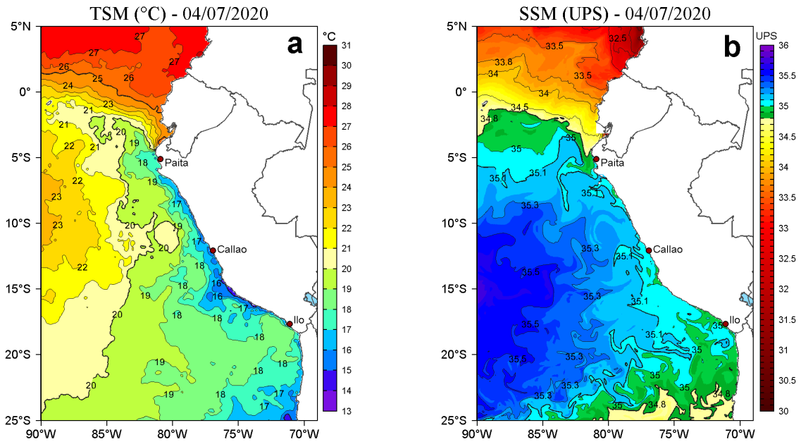
Figura 2. a) Temperatura superficial del mar (TSM, °C) y b) Salinidad superficial del mar (SSM, UPS), para el 04 de julio de 2020. Datos: OSTIA-UKMO-L4-GLOB-v2.0 (UK Met Office, 2012; Donlon et al, 2012) disponible en https://podaac.jpl.nasa.gov/dataset/OSTIA-UKMO-L4-GLOB-v2.0 para (a) y Hybrid Coordinate Ocean Model v. GOFS 3.1 (HYCOM; Halliwell et al., 1998; 2000; Bleck, 2001) para (b). Procesamiento: LHF/AFIOF/DGIOCC/IMARPE.
