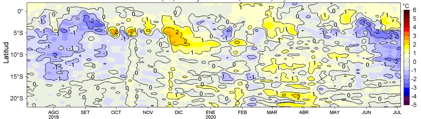
Figura 4. Variación promedio de las anomalías de la temperatura superficial del mar (TSM, °C) para una franja de 60 mn (~111 km) adyacente al litoral peruano para los últimos doce meses al 04 de julio de 2020. Datos: OSTIA-UKMO-L4-GLOB-v2.0 (UK Met. Office, 2012; Donlon et al, 2012) disponible en https://podaac.jpl.nasa.gov/dataset/OSTIA-UKMO-L4-GLOB-v2.0 . Las anomalías se calcularon con respecto al periodo 2007-2016. Procesamiento: LHF/AFIOF/DGIOCC/IMARPE.
