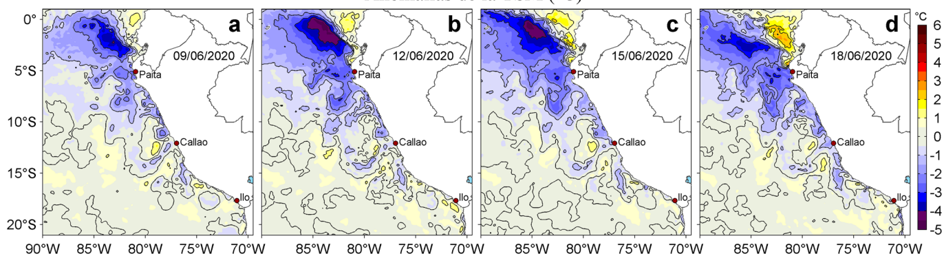
Figura 3. Anomalías de la temperatura superficial del mar (TSM, °C) para los días: a) 09, b) 12, c) 15 y d) 18 de junio de 2020. Las anomalías se calcularon respecto de la climatología para el periodo 2007-2016. Datos: OSTIA-UKMO-L4-GLOB-v2.0 (UK Met Office, 2012; Donlon et al, 2012). Procesamiento: LHFM/AFIOF/DGIOCC/IMARPE.
