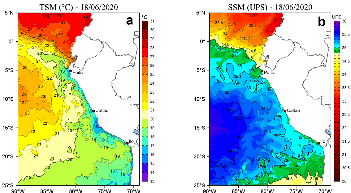
Figura 2. a) Temperatura superficial del mar (TSM, °C) y b) Salinidad superficial del mar (SSM, UPS), para el 18 de junio de 2020. Datos: OSTIA-UKMO-L4-GLOB-v2.0 (UK Met Office, 2012; Donlon et al, 2012) disponible en https://podaac.jpl.nasa.gov/dataset/OSTIA-UKMO-L4-GLOB-v2.0 para (a) y Hybrid Coordinate Ocean Model v. GOFS 3.1 (HYCOM; Halliwell et al., 1998; 2000; Bleck, 2001) para (b). Procesamiento: LHFM/AFIOF/DGIOCC/IMARPE.
