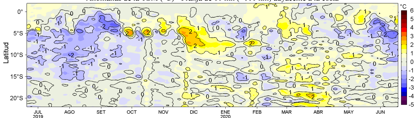
Figura 4. Variación promedio de las anomalías de la temperatura superficial del mar (TSM, °C) para una franja de 60 mn (~111 km) adyacente al litoral peruano para los últimos doce meses al 18 de junio de 2020. Datos: OSTIA-UKMO-L4-GLOB-v2.0 (UK Met. Office, 2012; Donlon et al, 2012) disponible en https://podaac.jpl.nasa.gov/dataset/OSTIA-UKMO-L4-GLOB-v2.0 . Las anomalías se calcularon con respecto al periodo 2007-2016. Procesamiento: LHFM/AFIOF/DGIOCC/IMARPE.
