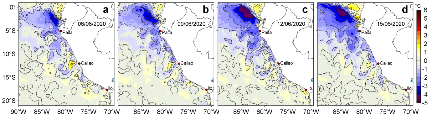
Figura 3. Anomalías de la temperatura superficial del mar (TSM, °C) para los días: a) 06, b) 09, c) 12 y d) 15 de junio de 2020. Las anomalías se calcularon respecto de la climatología para el periodo 2007-2016. Datos: OSTIA-UKMO-L4-GLOB-v2.0 (UK Met Office, 2012; Donlon et al, 2012). Procesamiento: LHFM/AFIOF/DGIOCC/IMARPE.
