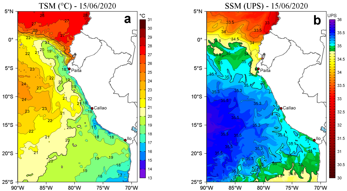
Figura 2. a) Temperatura superficial del mar (TSM, °C) y b) Salinidad superficial del mar (SSM, UPS), para el 15 de junio de 2020. Datos: OSTIA-UKMO-L4-GLOB-v2.0 (UK Met Office, 2012; Donlon et al, 2012) disponible en https://podaac.jpl.nasa.gov/dataset/OSTIA-UKMO-L4-GLOB-v2.0 para (a) y Hybrid Coordinate Ocean Model v. GOF3.1 (HYCOM; Halliwell et al., 1998; 2000; Bleck, 2001) para (b). Procesamiento: LHFM/AFIOF/DGIOCC/IMARPE.
