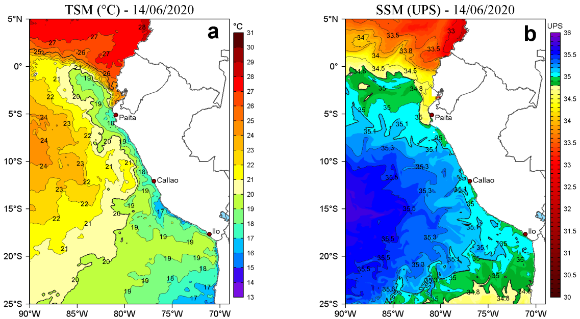
Figura 2. a) Temperatura superficial del mar (TSM, °C) y b) Salinidad superficial del mar (SSM, UPS), para el 14 de junio de 2020. Datos: OSTIA-UKMO-L4-GLOB-v2.0 (UK Met Office, 2012; Donlon et al, 2012) disponible en https://podaac.jpl.nasa.gov/dataset/OSTIA-UKMO-L4-GLOB-v2.0 para (a) y Hybrid Coordinate Ocean Model v. GOF3 3.1 (HYCOM; Halliwell et al., 1998; 2000; Bleck, 2001) para (b). Procesamiento: LHF/AFIOF/DGIOCC/IMARPE.
