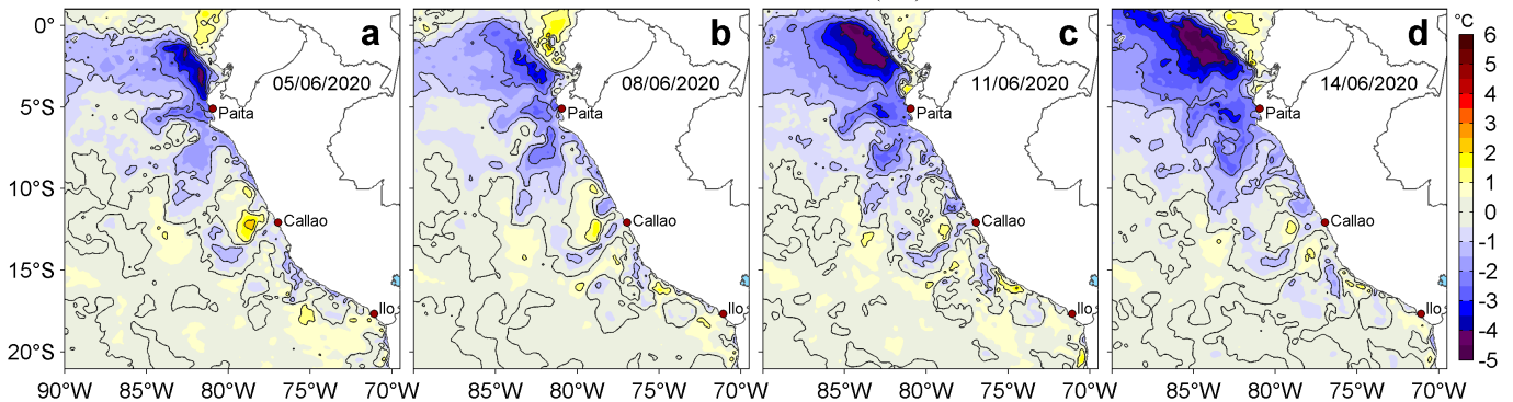
Figura 3. Anomalías de la temperatura superficial del mar (TSM, °C) para los días: a) 05, b) 08, c) 11 y d) 14 de junio de 2020. Las anomalías se calcularon respecto de la climatología para el periodo 2007-2016. Datos: OSTIA-UKMO-L4-GLOB-v2.0 (UK Met Office, 2012; Donlon et al, 2012). Procesamiento: LHF/AFIOF/DGIOCC/IMARPE.
