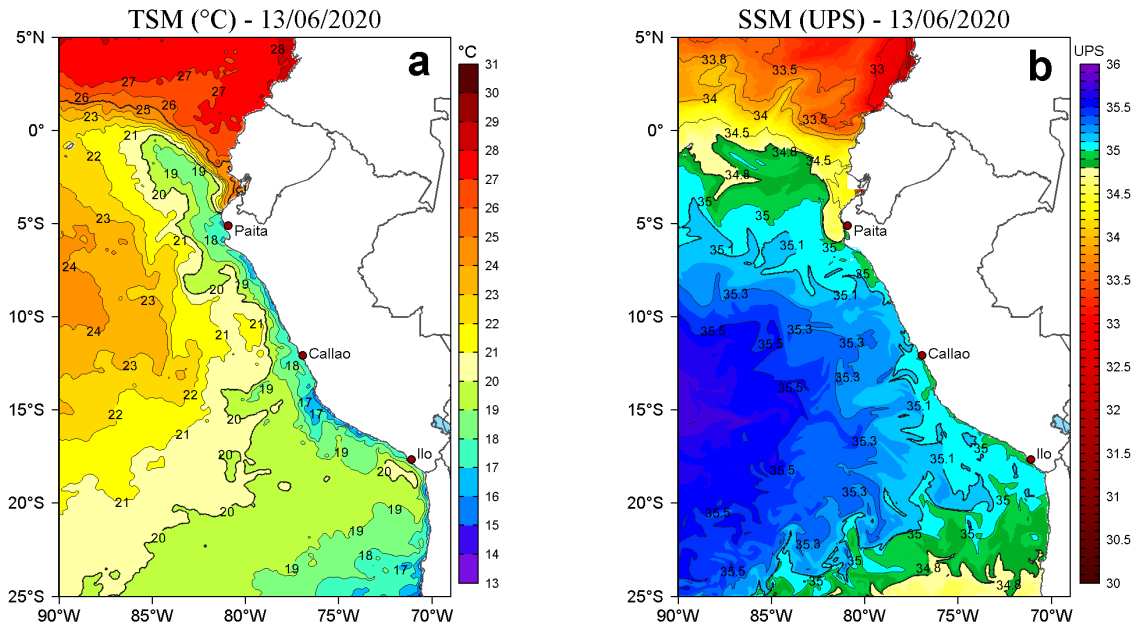
Figura 2. a) Temperatura superficial del mar (TSM, °C) y b) Salinidad superficial del mar (SSM, UPS), para el 13 de junio de 2020. Datos: OSTIA-UKMO-L4-GLOB-v2.0 (UK Met Office, 2012; Donlon et al, 2012) disponible en https://podaac.jpl.nasa.gov/dataset/OSTIA-UKMO-L4-GLOB-v2.0 para (a) y Hybrid Coordinate Ocean Model v. GOF3 3.1 (HYCOM; Halliwell et al., 1998; 2000; Bleck, 2001) para (b). Procesamiento: LHF/AFIOF/DGIOCC/IMARPE.
