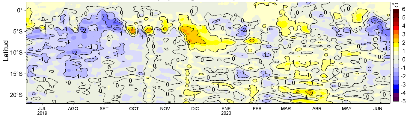
Figura 4. Variación promedio de las anomalías de la temperatura superficial del mar (TSM, °C) para una franja de 60 mn (~111 km) adyacente al litoral peruano para los últimos doce meses al 13 de junio de 2020. Datos: OSTIA-UKMO-L4-GLOB-v2.0 (UK Met. Office, 2012; Donlon et al, 2012) disponible en https://podaac.jpl.nasa.gov/dataset/OSTIA-UKMO-L4-GLOB-v2.0 . Las anomalías se calcularon con respecto al periodo 2007-2016. Procesamiento: LHF/AFIOF/DGIOCC/IMARPE.
