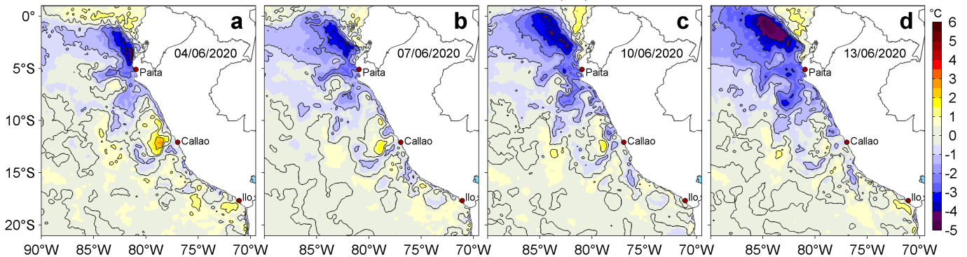
Figura 3. Anomalías de la temperatura superficial del mar (TSM, °C) para los días: a) 04, b) 07, c) 10 y d) 13 de junio de 2020. Las anomalías se calcularon respecto de la climatología para el periodo 2007-2016. Datos: OSTIA-UKMO-L4-GLOB-v2.0 (UK Met Office, 2012; Donlon et al, 2012). Procesamiento: LHF/AFIOF/DGIOCC/IMARPE.
