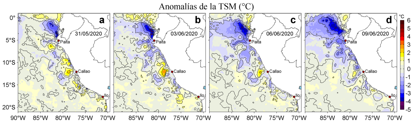
Figura 3. Anomalías de la temperatura superficial del mar (TSM, °C) para los días: a) 31 de mayo, b) 03, c) 06 y d) 09 de junio de 2020. Las anomalías se calcularon respecto de la climatología para el periodo 2007-2016. Datos: OSTIA-UKMO-L4-GLOB-v2.0 (UK Met Office, 2012; Donlon et al, 2012). Procesamiento: LHF/AFIOF/DGIOCC/IMARPE.
