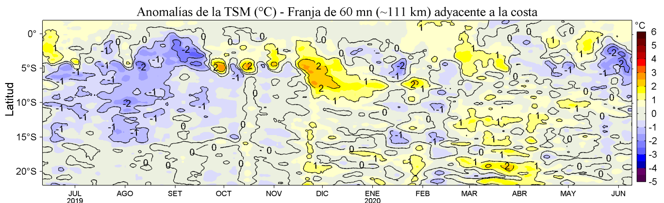
Figura 4. Variación promedio de las anomalías de la temperatura superficial del mar (TSM, °C) para una franja de 60 mn (~111 km) adyacente al litoral peruano para los últimos doce meses al 09 de junio de 2020. Datos: OSTIA-UKMO-L4-GLOB-v2.0 (UK Met. Office, 2012; Donlon et al, 2012) disponible en https://podaac.jpl.nasa.gov/dataset/OSTIA-UKMO-L4-GLOB-v2.0 . Las anomalías se calcularon con respecto al periodo 2007-2016. Procesamiento: LHF/AFIOF/DGIOCC/IMARPE.
