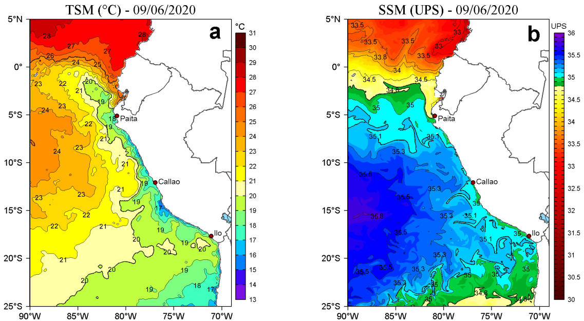
Figura 2. a) Temperatura superficial del mar (TSM, °C) y b) Salinidad superficial del mar (SSM, UPS), para el 09 de junio de 2020. Datos: OSTIA-UKMO-L4-GLOB-v2.0 (UK Met Office, 2012; Donlon et al, 2012) disponible en https://podaac.jpl.nasa.gov/dataset/OSTIA-UKMO-L4-GLOB-v2.0 para (a) y Hybrid Coordinate Ocean Model v. GOFS 3.1 (HYCOM; Halliwell et al., 1998; 2000; Bleck, 2001) para (b). Procesamiento: LHF/AFIOF/DGIOCC/IMARPE.
