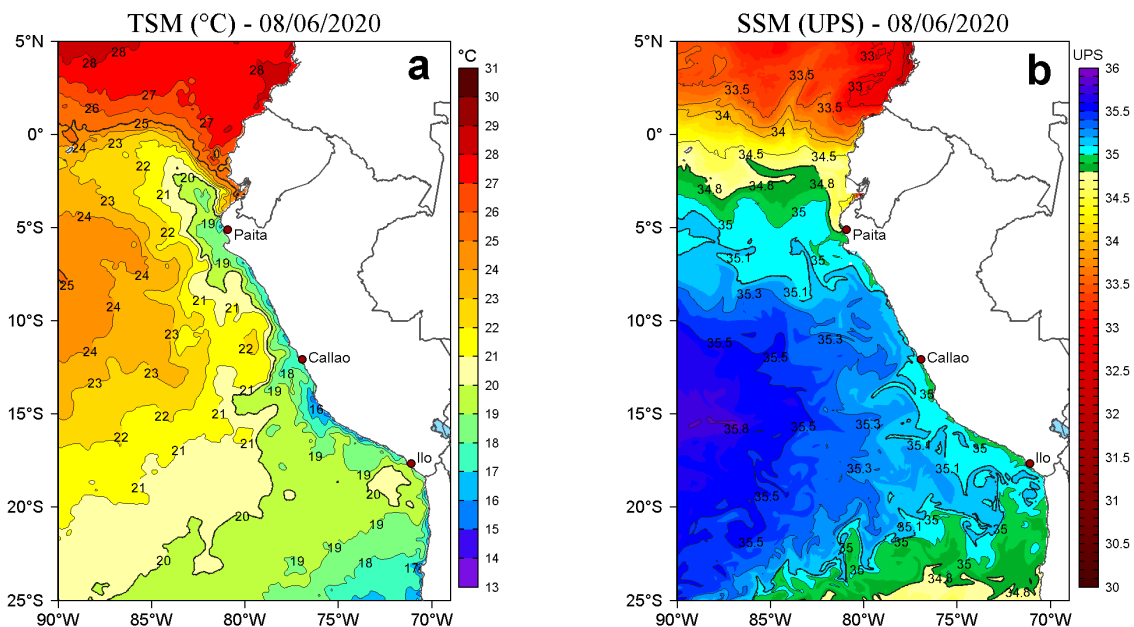
Figura 2. a) Temperatura superficial del mar (TSM, °C) y b) Salinidad superficial del mar (SSM, UPS), para el 08 de junio de 2020. Datos: OSTIA-UKMO-L4-GLOB-v2.0 (UK Met Office, 2012; Donlon et al, 2012) disponible en https://podaac.jpl.nasa.gov/dataset/OSTIA-UKMO-L4-GLOB-v2.0 para (a) y Hybrid Coordinate Ocean Model v. GOFS 3.1 (HYCOM; Halliwell et al., 1998; 2000; Bleck, 2001) para (b). Procesamiento: LHF/AFIOF/DGIOCC/IMARPE.
