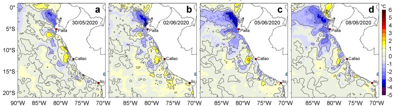
Figura 3. Anomalías de la temperatura superficial del mar (TSM, °C) para los días: a) 30 de mayo, b) 02, c) 05 y d) 08 de junio de 2020. Las anomalías se calcularon respecto de la climatología para el periodo 2007-2016. Datos: OSTIA-UKMO-L4-GLOB-v2.0 (UK Met Office, 2012; Donlon et al, 2012). Procesamiento: LHF/AFIOF/DGIOCC/IMARPE.
