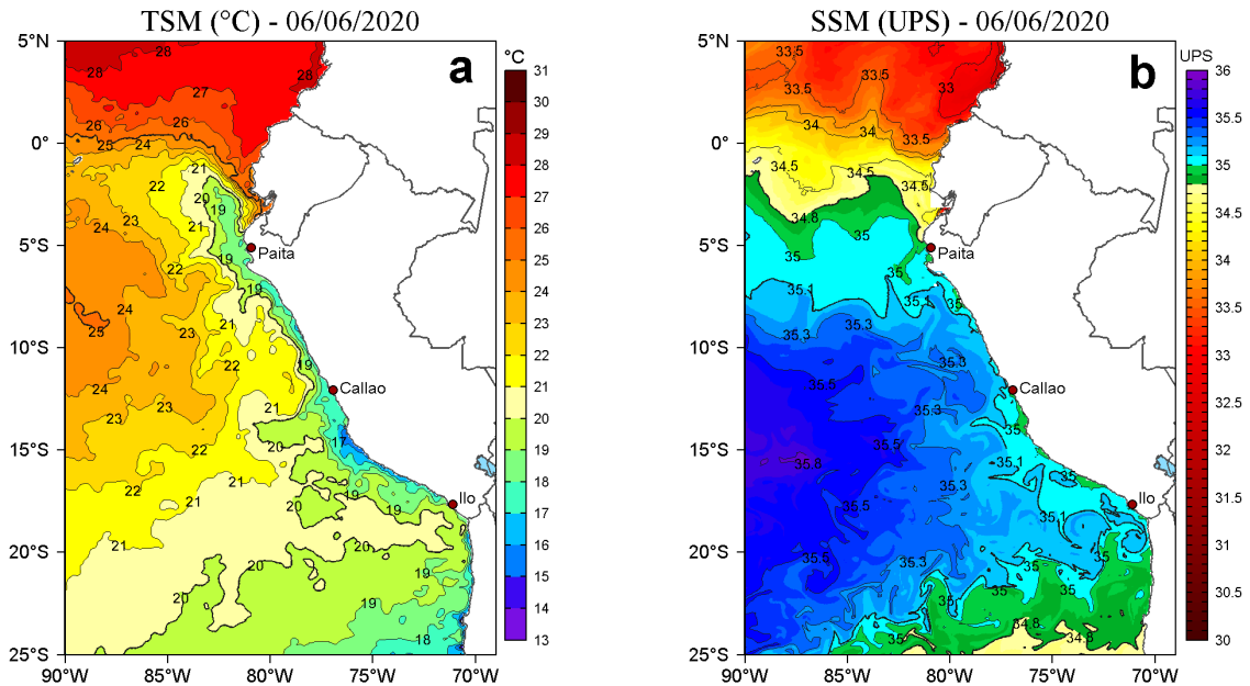
Figura 2. a) Temperatura superficial del mar (TSM, °C) y b) Salinidad superficial del mar (SSM, UPS), para el 06 de junio de 2020. Datos: OSTIA-UKMO-L4-GLOB-v2.0 (UK Met Office, 2012; Donlon et al, 2012) disponible en https://podaac.jpl.nasa.gov/dataset/OSTIA-UKMO-L4-GLOB-v2.0 para (a) y Hybrid Coordinate Ocean Model v. GOFS 3.1 (HYCOM; Halliwell et al., 1998; 2000; Bleck, 2001) para (b). Procesamiento: LHFM/AFIOF/DGIOCC/IMARPE.
