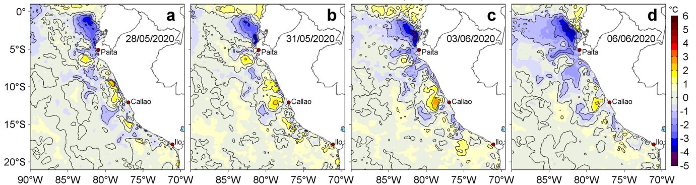
Figura 3. Anomalías de la temperatura superficial del mar (TSM, °C) para los días: a) 28 y b) 31 de mayo, c) 03 y d) 06 de junio de 2020. Las anomalías se calcularon respecto de la climatología para el periodo 2007-2016. Datos: OSTIA-UKMO-L4-GLOB-v2.0 (UK Met Office, 2012; Donlon et al, 2012). Procesamiento: LHFM/AFIOF/DGIOCC/IMARPE.
