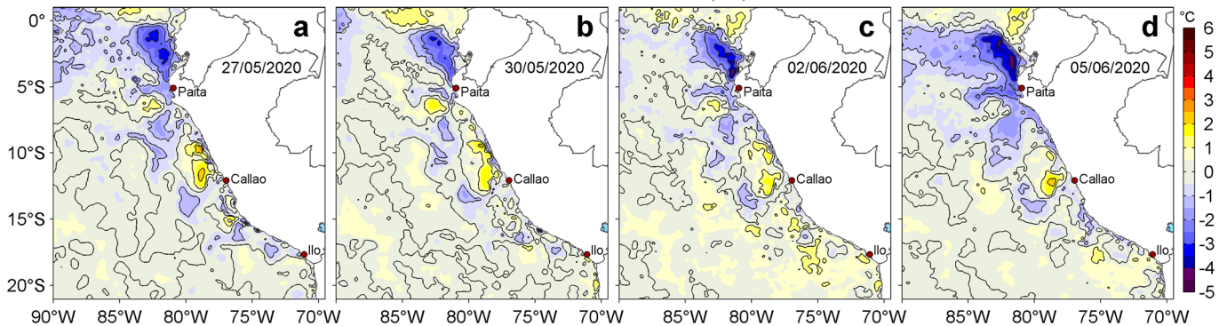
Figura 3. Anomalías de la temperatura superficial del mar (TSM, °C) para los días: a) 27 y b) 30 de mayo, c) 02 y d) 05 de junio de 2020. Las anomalías se calcularon respecto de la climatología para el periodo 2007-2016. Datos: OSTIA-UKMO-L4-GLOB-v2.0 (UK Met Office, 2012; Donlon et al, 2012). Procesamiento: LHF/AFIOF/DGIOCC/IMARPE.
