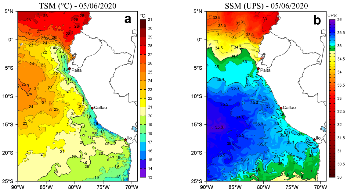
Figura 2. a) Temperatura superficial del mar (TSM, °C) y b) Salinidad superficial del mar (SSM, UPS), para el 05 de junio de 2020. Datos: OSTIA-UKMO-L4-GLOB-v2.0 (UK Met Office, 2012; Donlon et al, 2012) disponible en https://podaac.jpl.nasa.gov/dataset/OSTIA-UKMO-L4-GLOB-v2.0 para (a) y Hybrid Coordinate Ocean Model v. GOFS 3.1 (HYCOM; Halliwell et al., 1998; 2000; Bleck, 2001) para (b). Procesamiento: LHF/AFIOF/DGIOCC/IMARPE.
