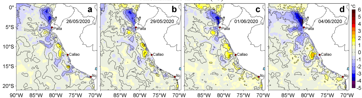
Figura 3. Anomalías de la temperatura superficial del mar (TSM, °C) para los días: a) 26 y b) 29 de mayo, c) 01 y d) 04 de junio de 2020. Las anomalías se calcularon respecto de la climatología para el periodo 2007-2016. Datos: OSTIA-UKMO-L4-GLOB-v2.0 (UK Met Office, 2012; Donlon et al, 2012). Procesamiento: LHFm/AFIOF/DGIOCC/IMARPE.
