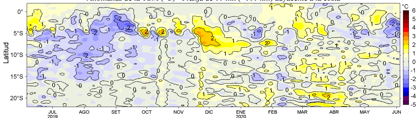
Figura 4. Variación promedio de las anomalías de la temperatura superficial del mar (TSM, °C) para una franja de 60 mn (~111 km) adyacente al litoral peruano para los últimos doce meses al 04 de junio de 2020. Datos: OSTIA-UKMO-L4-GLOB-v2.0 (UK Met. Office, 2012; Donlon et al, 2012) disponible en https://podaac.jpl.nasa.gov/dataset/OSTIA-UKMO-L4-GLOB-v2.0 . Las anomalías se calcularon con respecto al periodo 2007-2016. Procesamiento: LHFm/AFIOF/DGIOCC/IMARPE.
