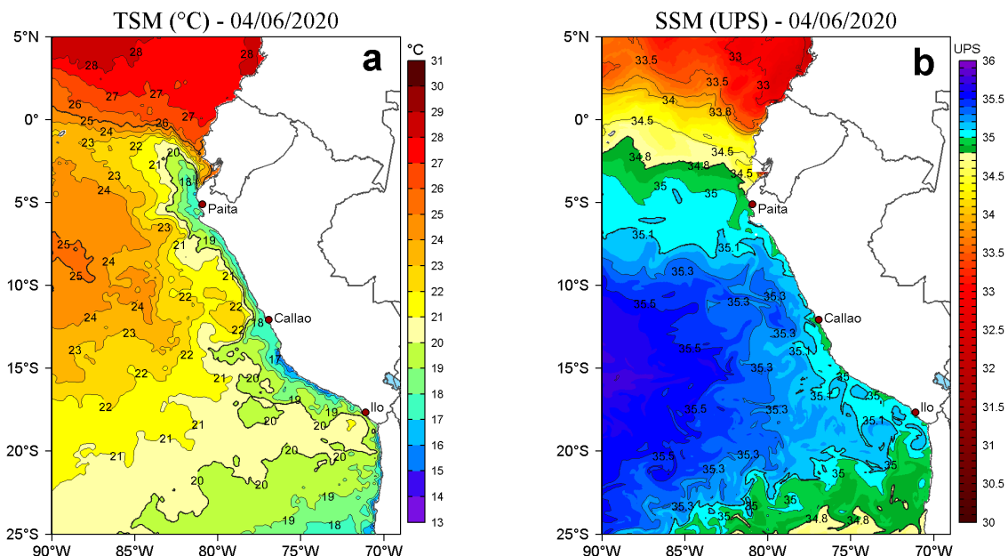
Figura 2. a) Temperatura superficial del mar (TSM, °C) y b) Salinidad superficial del mar (SSM, UPS), para el 04 de junio de 2020. Datos: OSTIA-UKMO-L4-GLOB-v2.0 (UK Met Office, 2012; Donlon et al, 2012) disponible en https://podaac.jpl.nasa.gov/dataset/OSTIA-UKMO-L4-GLOB-v2.0 para (a) y Hybrid Coordinate Ocean Model v. GOFS 3.1 (HYCOM; Halliwell et al., 1998; 2000; Bleck, 2001) para (b). Procesamiento: LHFm/AFIOF/DGIOCC/IMARPE.
