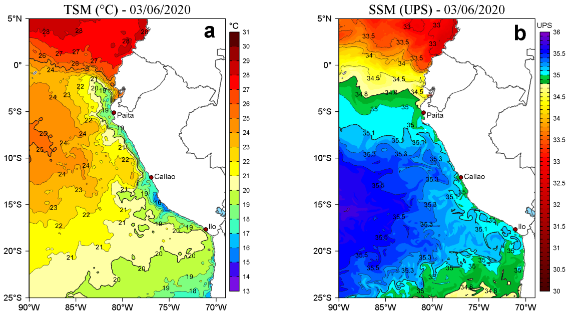
Figura 2. a) Temperatura superficial del mar (TSM, °C) y b) Salinidad superficial del mar (SSM, UPS), para el 03 de junio de 2020. Datos: OSTIA-UKMO-L4-GLOB-v2.0 (UK Met Office, 2012; Donlon et al, 2012) disponible en https://podaac.jpl.nasa.gov/dataset/OSTIA-UKMO-L4-GLOB-v2.0 para (a) y Hybrid Coordinate Ocean Model v. GOFS 3.1 (HYCOM; Halliwell et al., 1998; 2000; Bleck, 2001) para (b). Procesamiento: LHFm/AFIOF/DGIOCC/IMARPE.
