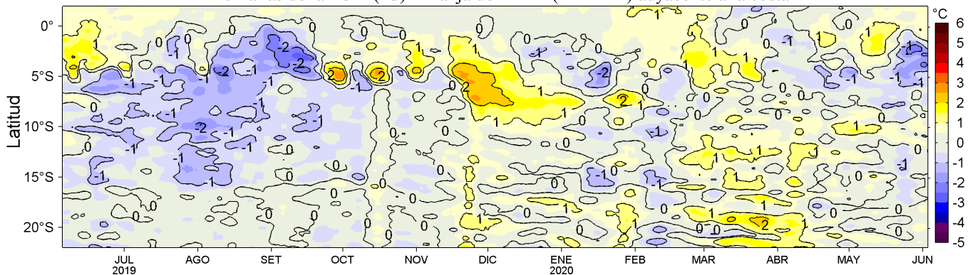
Figura 4. Variación promedio de las anomalías de la temperatura superficial del mar (TSM, °C) para una franja de 60 mn (~111 km) adyacente al litoral peruano para los últimos doce meses al 03 de junio de 2020. Datos: OSTIA-UKMO-L4-GLOB-v2.0 (UK Met. Office, 2012; Donlon et al, 2012) disponible en https://podaac.jpl.nasa.gov/dataset/OSTIA-UKMO-L4-GLOB-v2.0 . Las anomalías se calcularon con respecto al periodo 2007-2016. Procesamiento: LHFm/AFIOF/DGIOCC/IMARPE.
