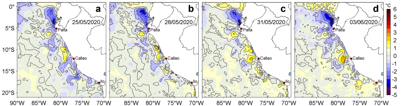
Figura 3. Anomalías de la temperatura superficial del mar (TSM, °C) para los días: a) 25, b) 28 y c) 31 de mayo y d) 03 de junio de 2020. Las anomalías se calcularon respecto de la climatología para el periodo 2007-2016. Datos: OSTIA-UKMO-L4-GLOB-v2.0 (UK Met Office, 2012; Donlon et al, 2012). Procesamiento: LHFm/AFIOF/DGIOCC/IMARPE.
