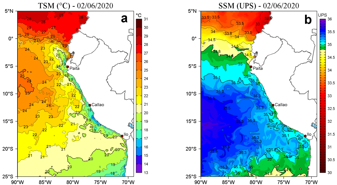
Figura 2. a) Temperatura superficial del mar (TSM, °C) y b) Salinidad superficial del mar (SSM, UPS), para el 02 de junio de 2020. Datos: OSTIA-UKMO-L4-GLOB-v2.0 (UK Met Office, 2012; Donlon et al, 2012) disponible en https://podaac.jpl.nasa.gov/dataset/OSTIA-UKMO-L4-GLOB-v2.0 para (a) y Hybrid Coordinate Ocean Model v. GOFS 3.1 (HYCOM; Halliwell et al., 1998; 2000; Bleck, 2001) para (b). Procesamiento: LHFm/AFIOF/DGIOCC/IMARPE.
