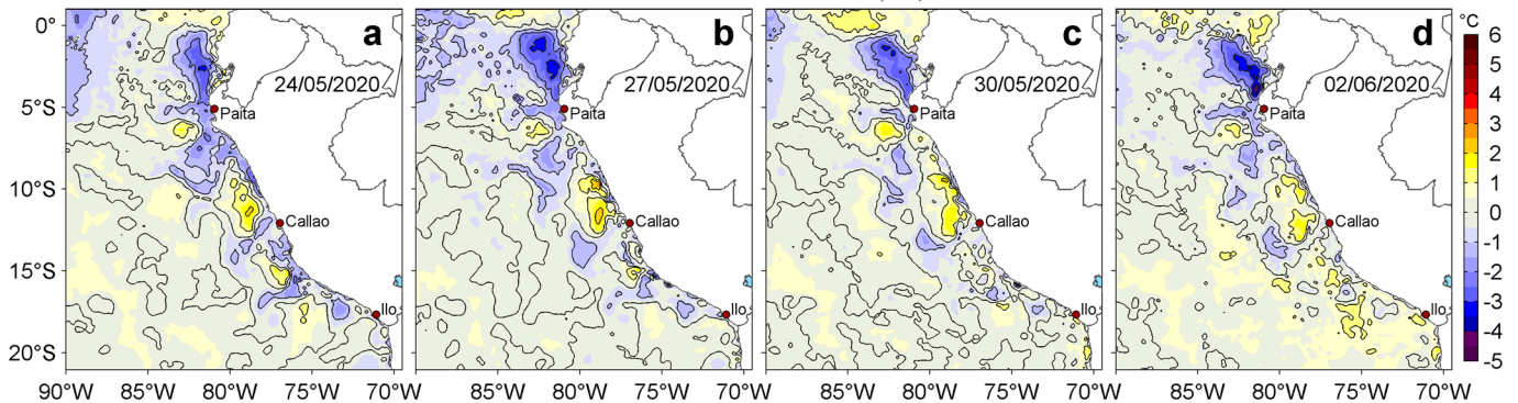
Figura 3. Anomalías de la temperatura superficial del mar (TSM, °C) para los días: a) 24, b) 27 y c) 30 de mayo y d) 02 de junio de 2020. Las anomalías se calcularon respecto de la climatología para el periodo 2007-2016. Datos: OSTIA-UKMO-L4-GLOB-v2.0 (UK Met Office, 2012; Donlon et al, 2012). Procesamiento: LHFm/AFIOF/DGIOCC/IMARPE.
